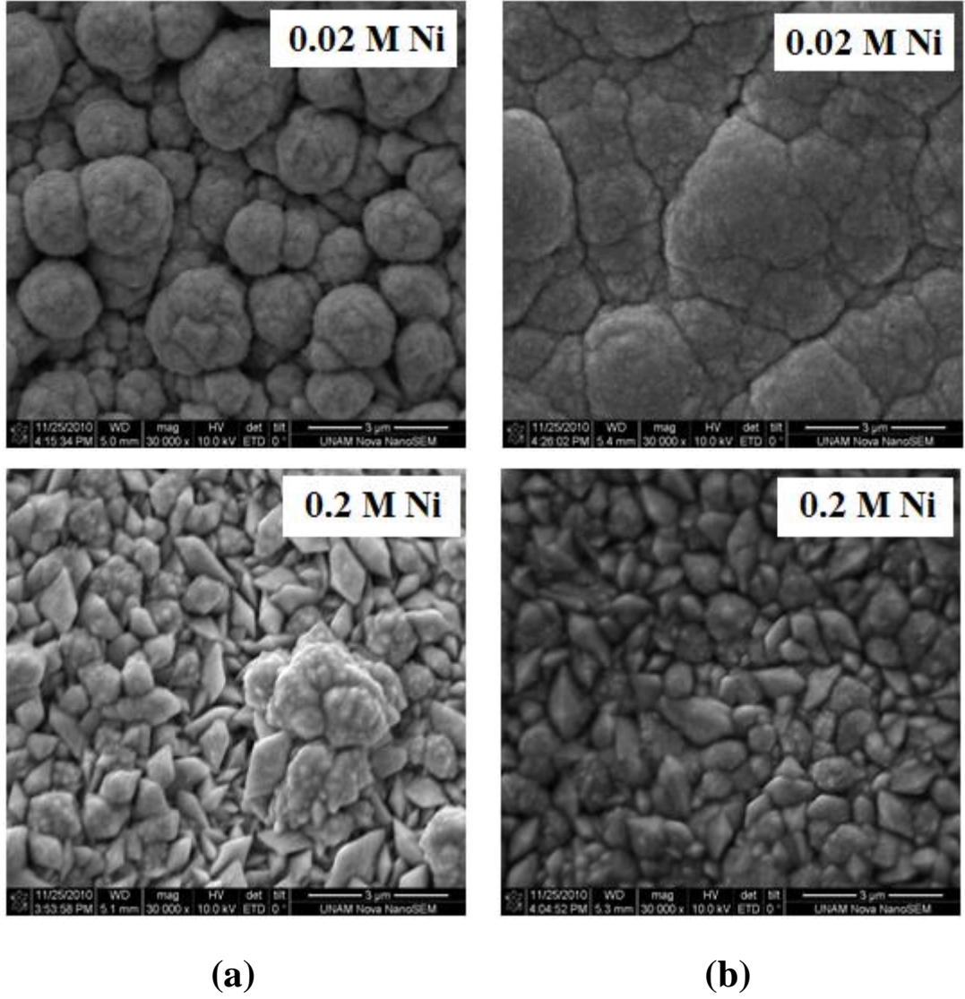
Şekil 4.8. 0.02M Ni ve 0.2M Ni içeren çözeltilerden büyütülen (a) 600[CoNi(4nm)/Cu(1nm)], (b) 429[CoNi(4nm)/Cu(3nm)] süperörgülerinin SEM görüntüleri
