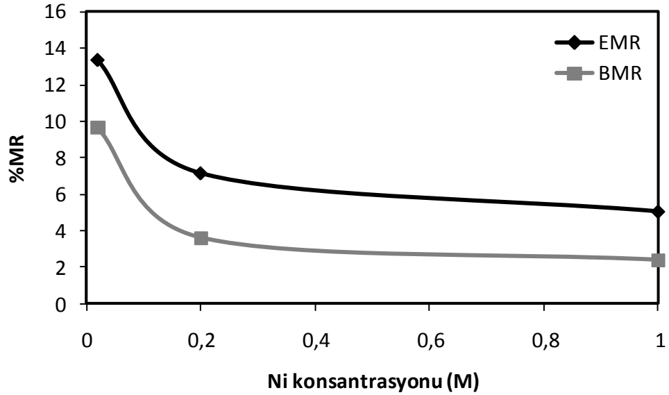
Şekil 4.22. 667 [CoNi (4 nm)/ Cu (0.5 nm)] süperörgülerinin EMR ve BMR değerlerinin Ni konsantrasyonuna bağlı değişimi
