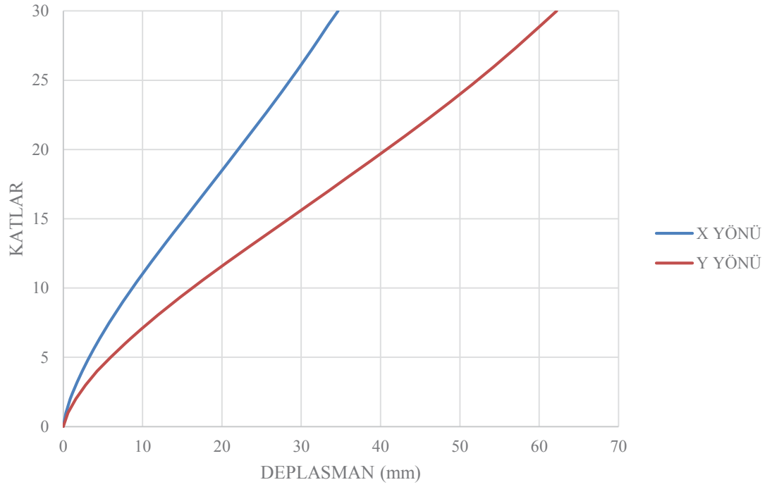
Şekil 4.7. Rüzgar hesabı maksimum kat deplasmanları
