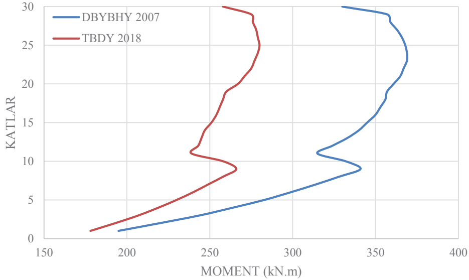
Şekil 4.54. B57 kirişi moment değerleri
