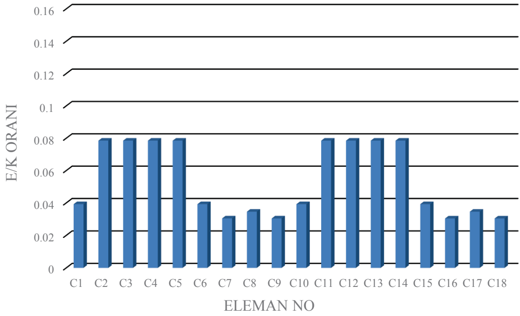
Şekil 4.36. 20. kat kolon kesme kuvveti E/K oranları
