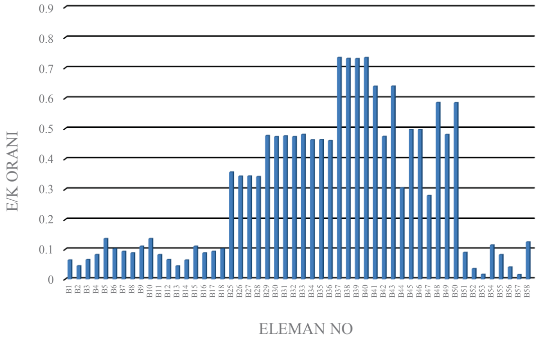
Şekil 4.29. 30. kat kirişlerinin moment E/K oranları
