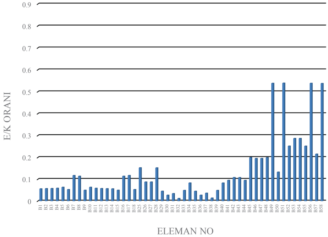
Şekil 4.26. 1. kat kirişlerinin moment E/K oranları
