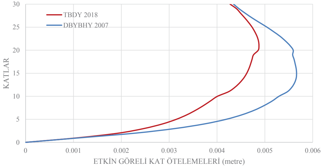
Şekil 4.45. Y yönü etkin görelî kat ötelemelerinin karşılaştırması
