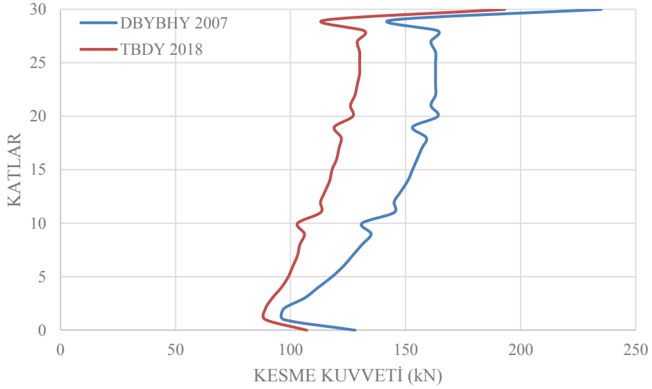
Şekil 4.48. C17 kolonu kesme kuvveti değerleri
