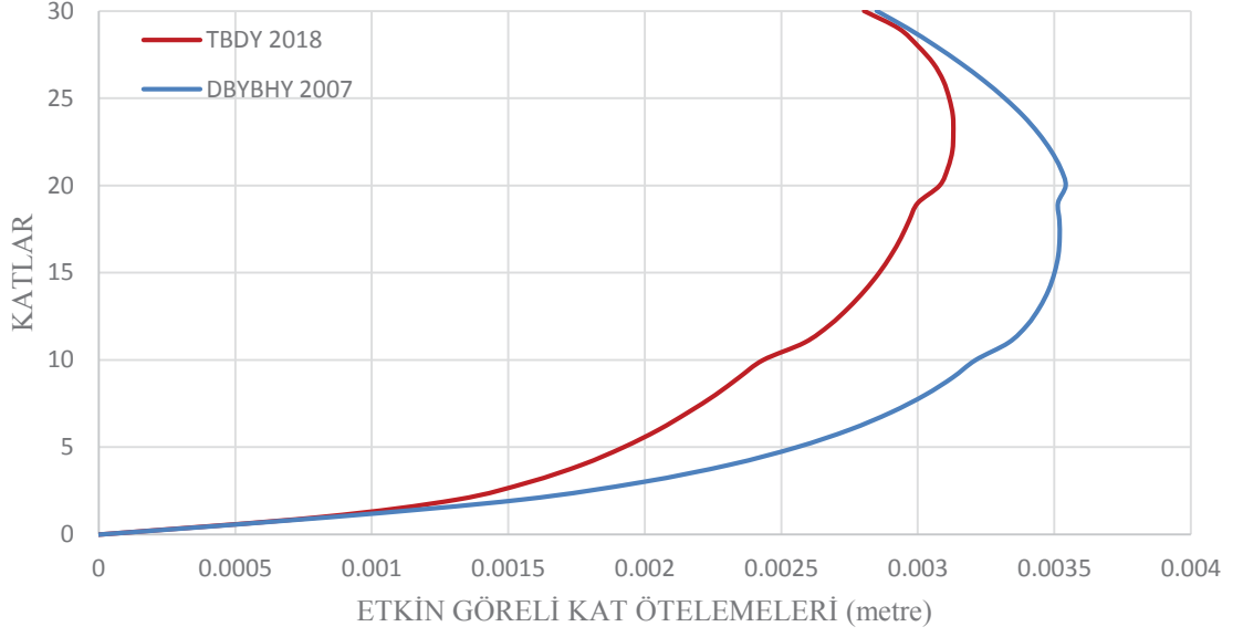
Şekil 4.44. X yönü etkin görelî kat ötelemelerinin karşılaştırması
