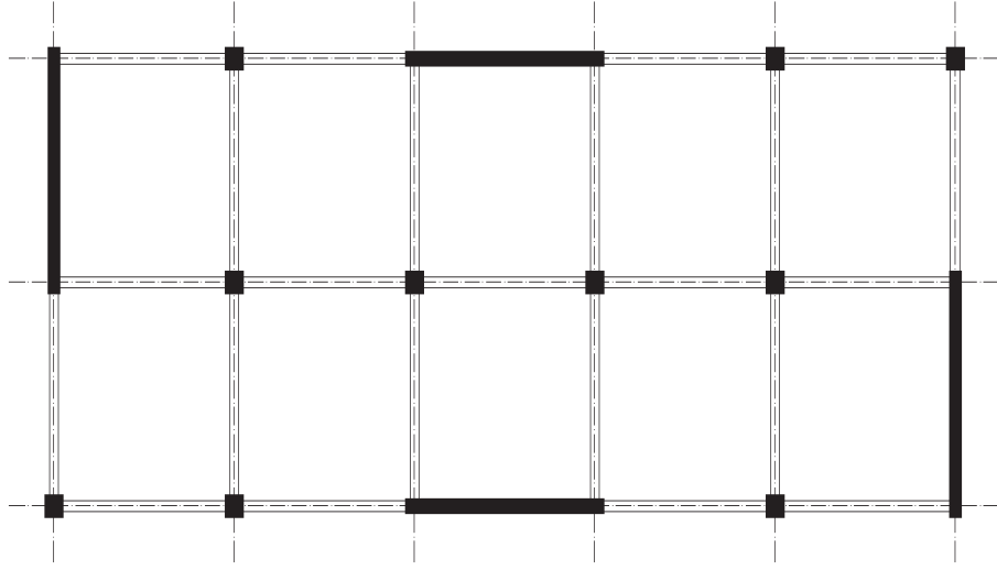
Şekil 2.4. Perde ve çerçevden oluşan sistem
