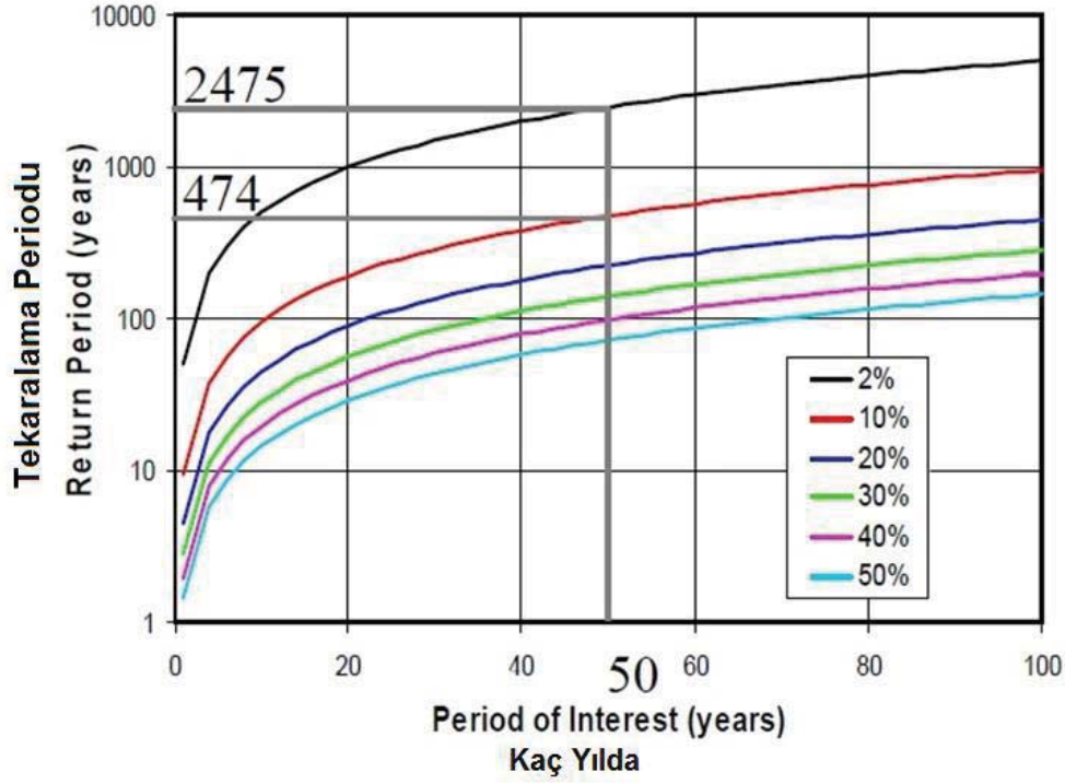
Şekil 3.1. Deprem yer hareketi tekraralama periyodu
