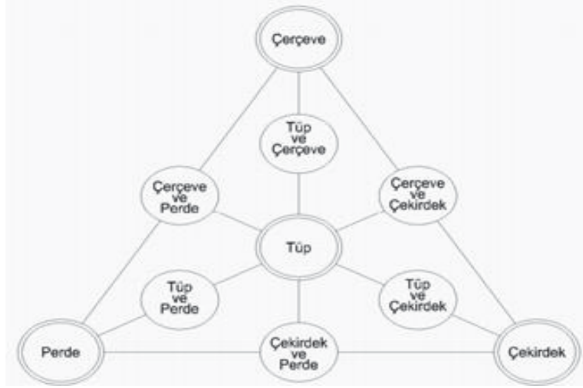
Şekil 2.2. Yüksek yapıların taşıyıcı sistemlerinin sınıflandırılması (Drosdov ve Lishak 1978)
