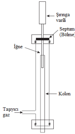
Şekil 2.6. Enjeksiyon bölmesinin kesiti (Harvey 1996)
