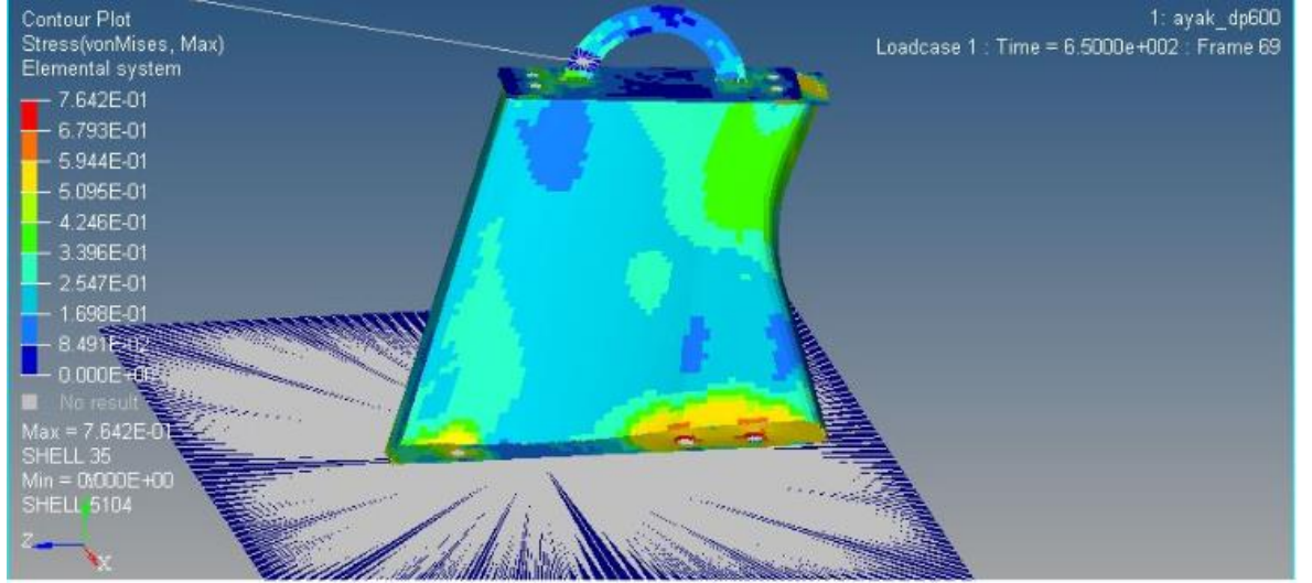
Şekil 4.15. DP600 3 mm-Von-mises gerilmesi
