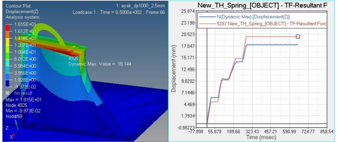
Şekil 4.28. DP1000 – 2,5 mm ayak için kuvvet-yer değişimi-zaman grafiği
