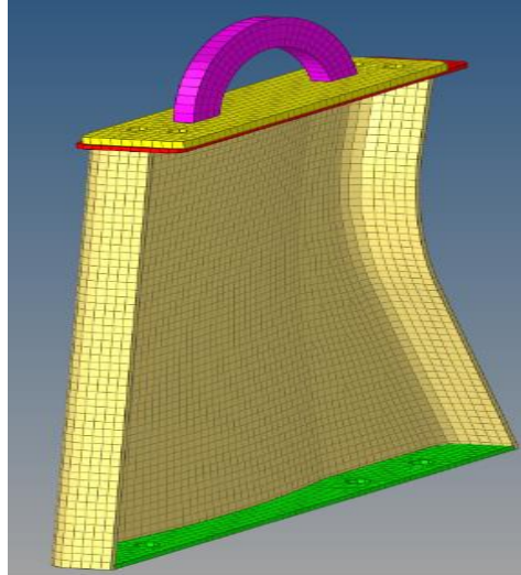
Şekil 3.3 Ayak ve aparatın genel mesh yapısı
