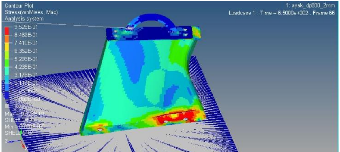
Şekil 4.23. DP800 2 mm-Von-mises gerilmesi
