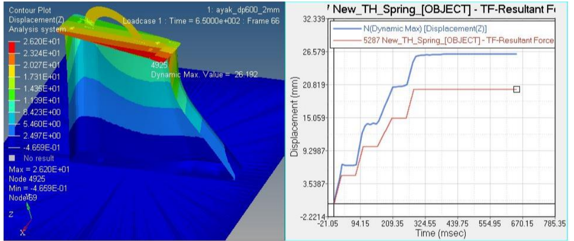
Şekil 4.16. DP600-2 mm ayak için kuvvet-yer değişimi-zaman grafiği
