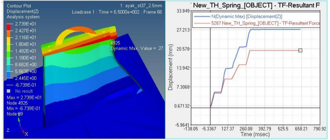
Şekil 4.4. St37-2,5 mm ayak için kuvvet-yer değişimi-zaman grafiği
