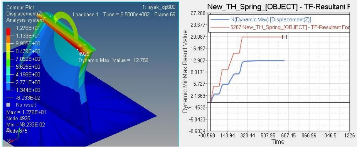
Şekil 4.14. DP600-3 mm ayak için kuvvet-yer değişimi-zaman grafiği
