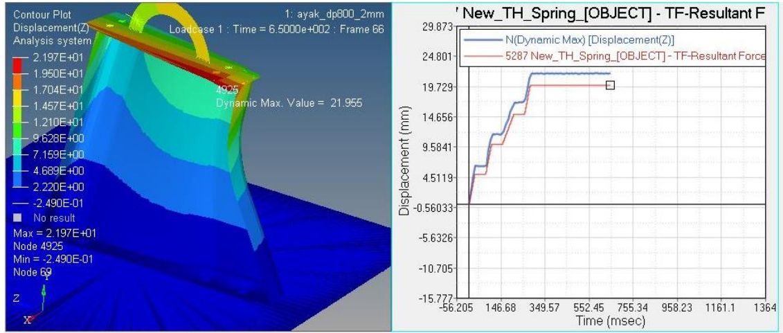
Şekil 4.22. DP800 - 2 mm ayak için kuvvet-yer değişimi-zaman grafiği
