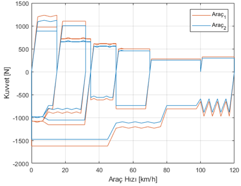
Şekil 41: NEDC Test-Araç.1 ve Araç.2 Kuvvet-Hız Haritası
