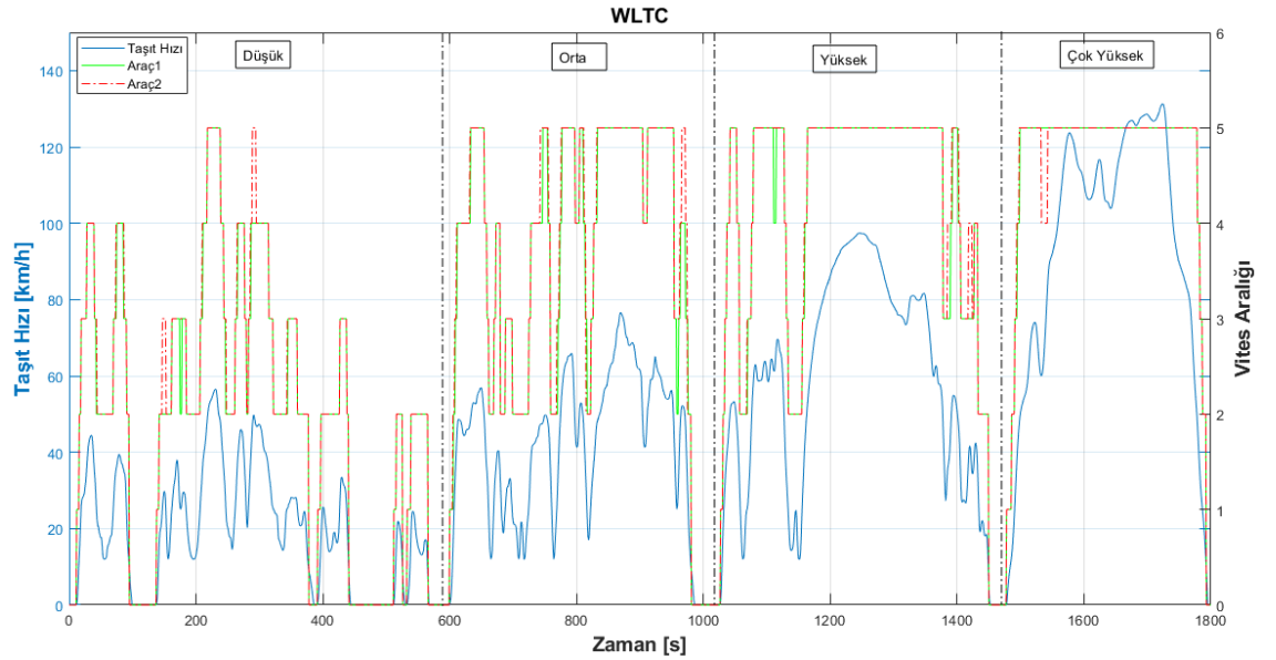
Şekil 14: WLTC Hız Profili ve Vites Aralığı
