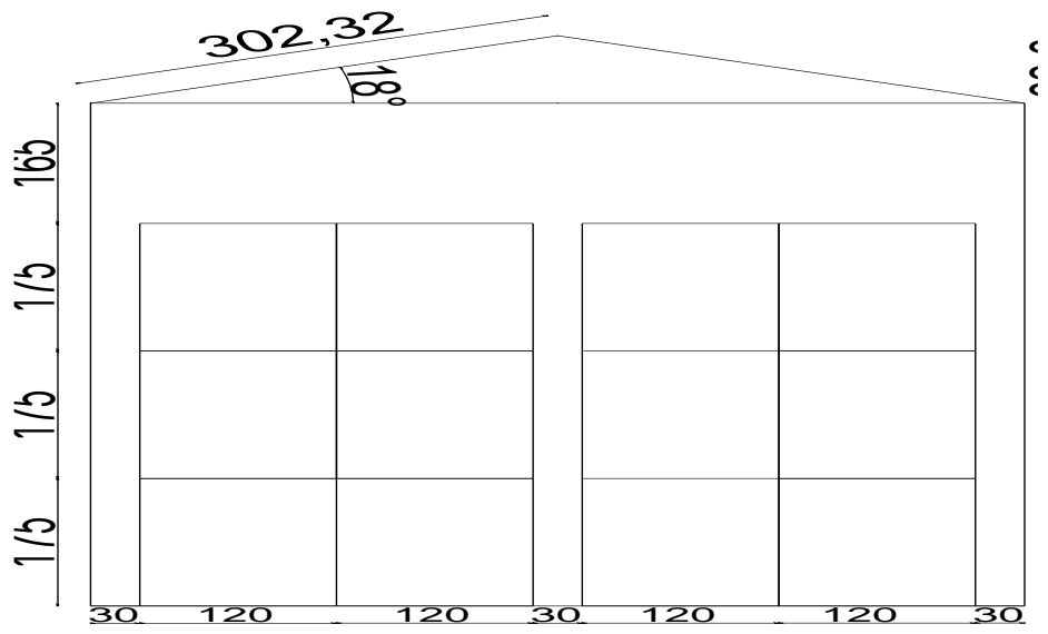
100 ton armut depolama kapasitesine sahip soğuk oda en kesiti
