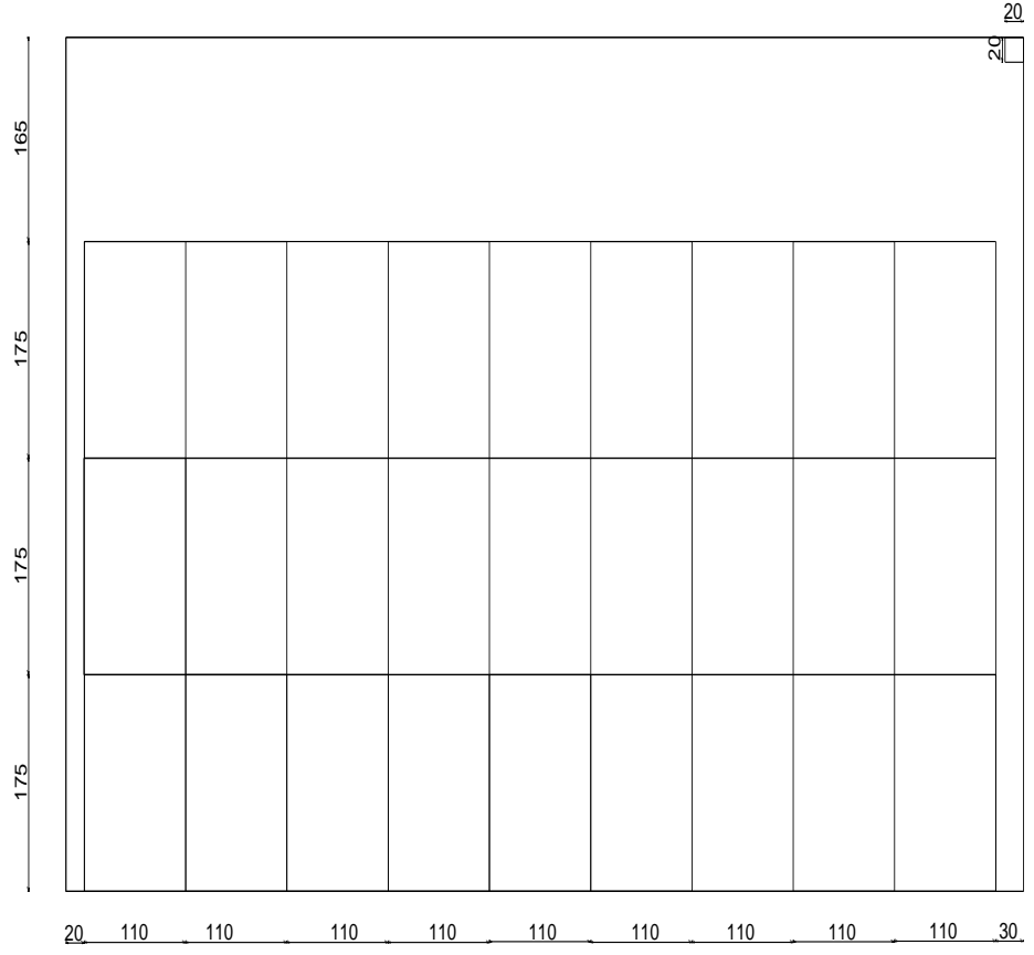
50 ton armut depolama kapasitesine sahip soğuk oda boy kesiti
