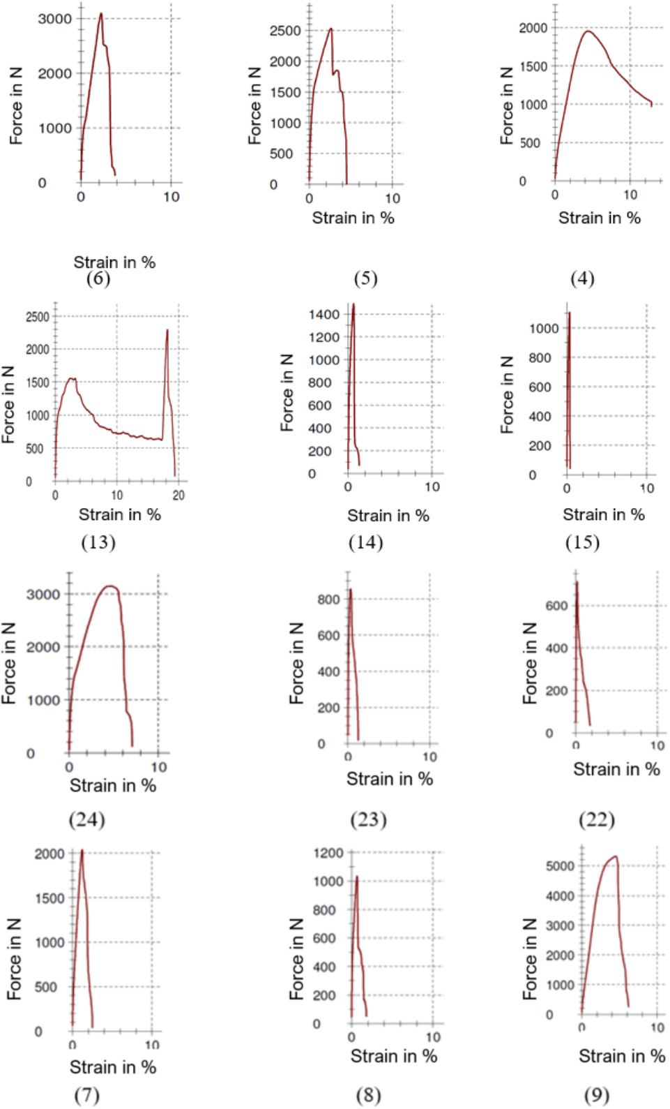
Şekil 4.2. Sabit laser gücünde ve odak mesafesinde farklı kaynak hızları ile birleştirilen numunelerin çekme testi sonucunda elde edilen eğrileri
