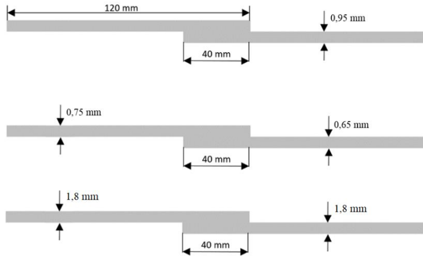
Şekil 3.2. Numune boyutları
