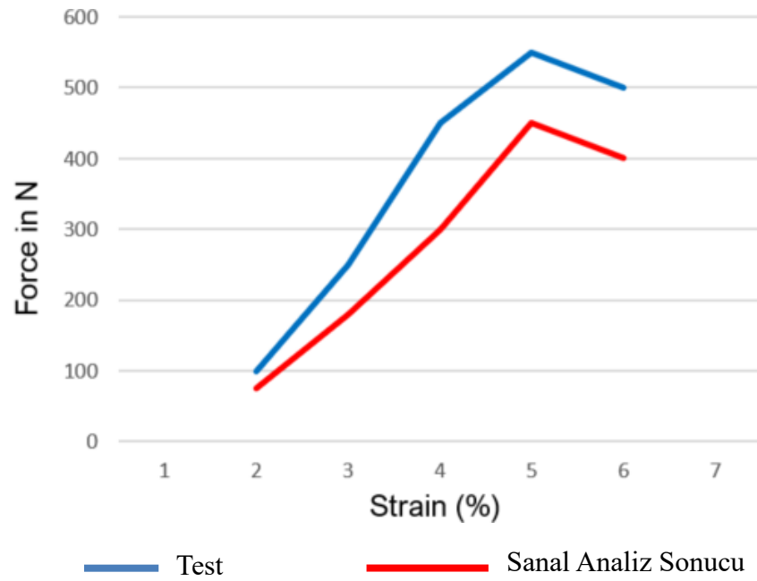
Şekil 4.36. Gerçek ve sanal test sonuçlarının kıyaslanması
