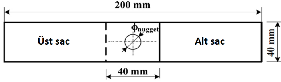
Şekil 3.7. Çekme test numune ölçüleri
