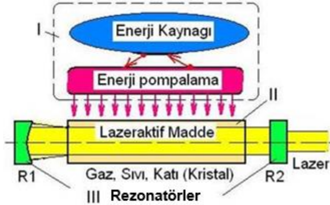
Şekil 2.4. Laser ışınının oluşumunda kullanılan ekipmanların şematik görüntüsü (Kakaçoğlu 2014)
