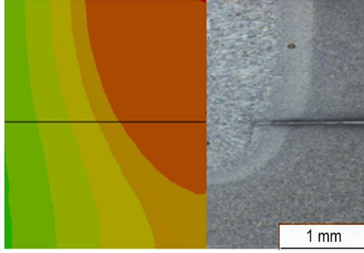
Şekil 4.33. Kaynak kesit görüntüsü ile sonlu elemanlar analiz sonucunun karşılaştırması (Ansys)
