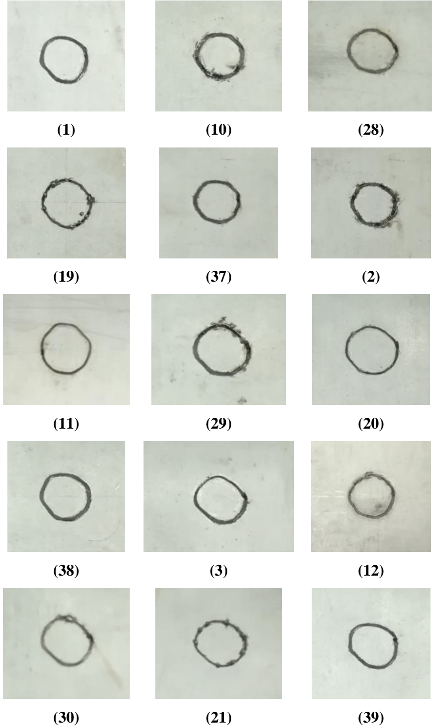
Şekil 4.5. Sabit laser gücünde ve kaynak hızında farklı odak mesafelerinde birleştirilen numunelerin görüntüleri
