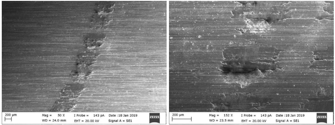
Şekil 4.9. Plazma nitrülenmemiş D2 takım çeliğinin SEM fotoğrafı (a) plazma nitrülenmiş D2 takım çeliğinin SEM fotoğrafı (b)
