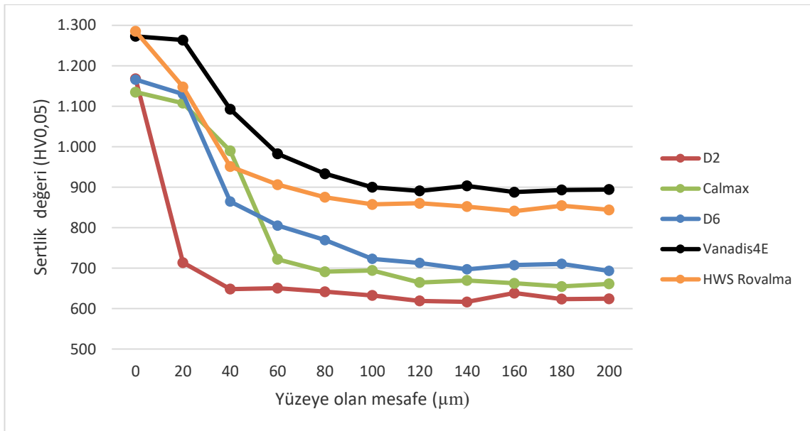
Şekil 4.3. Kesitten derine mikrosertlik dağılımı
