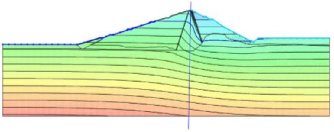
Şekil 2.5. İkizdere Barajı k=2,43 \times 10^{-8} m/s için sızma analizi (Çelik 2014)
