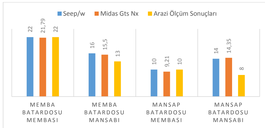
Şekil 4.10. Analizler ve arazi ölçümleri sonucu elde edilen toplam yüklerle ait karşılaştırma
