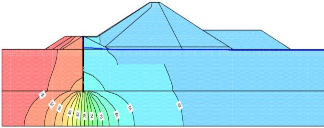
Şekil 2.4. Muratlı Barajı'na ait sızma analizi (Ünsever 2007)
