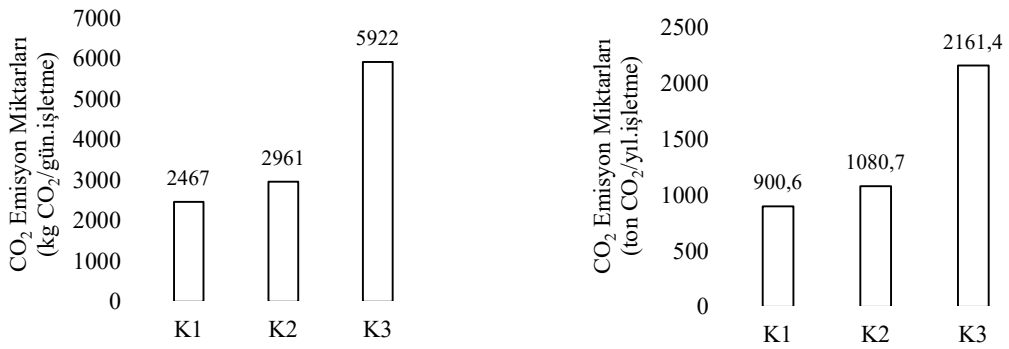
Şekil 4.5. Broylardan kaynaklanan CO 2 emisyonları
