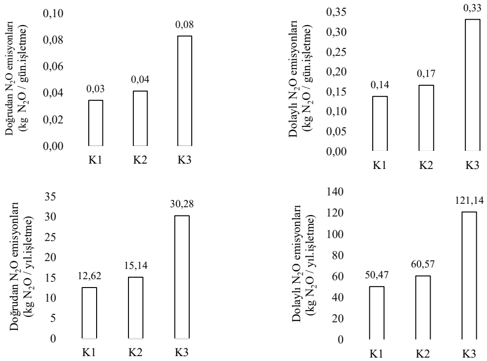
Şekil 4.3. İşletmelerin doğrudan ve dolaylı N 2 O emisyonları
