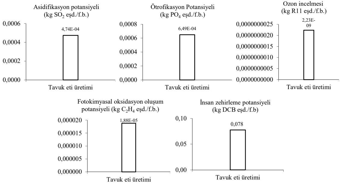
Şekil 4.11. K3 fonksiyonel birim başına çevresel etkiler
