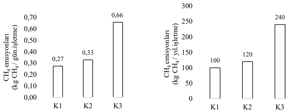
Şekil 4.4. CH 4 emisyonları
