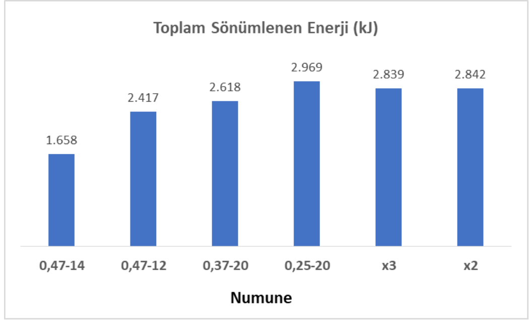
Şekil 4.4. Çarpışma kutularının sönümledikleri enerji miktarları
