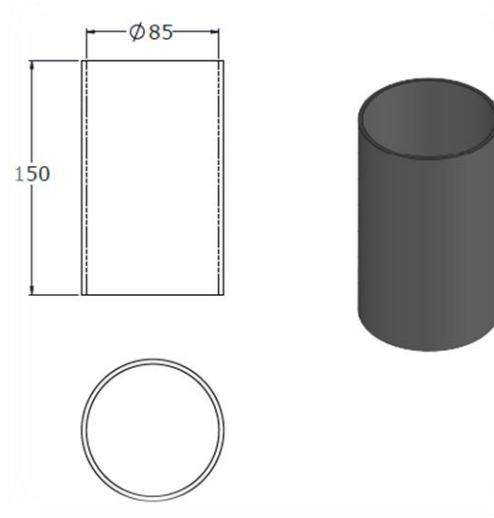
Şekil 3.2. Çarpışma kutusunun boyutları
