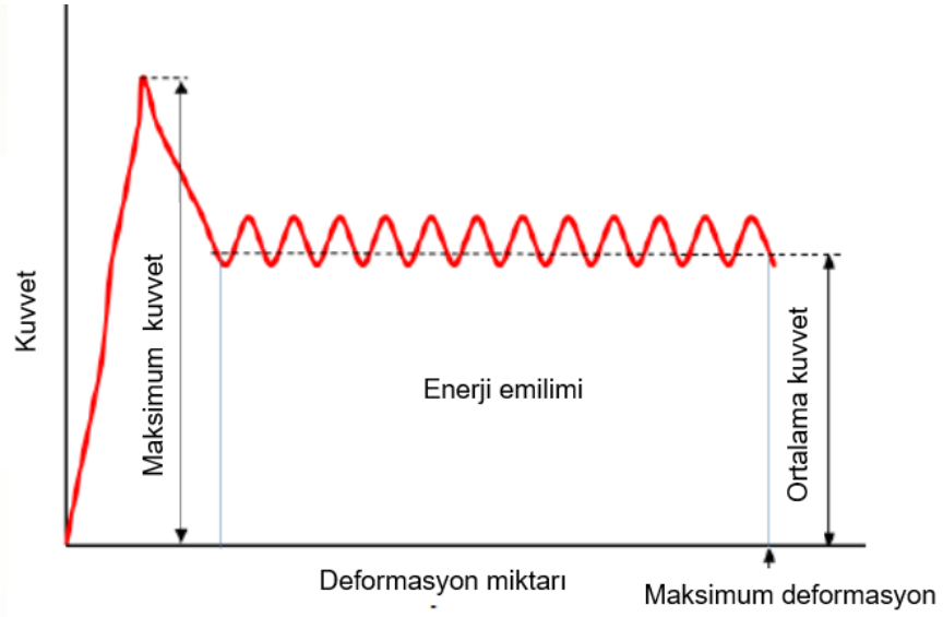
Şekil 2.1. İdeal bir çarpışma kutusunun Kuvvet-Deformasyon miktarı grafiği
