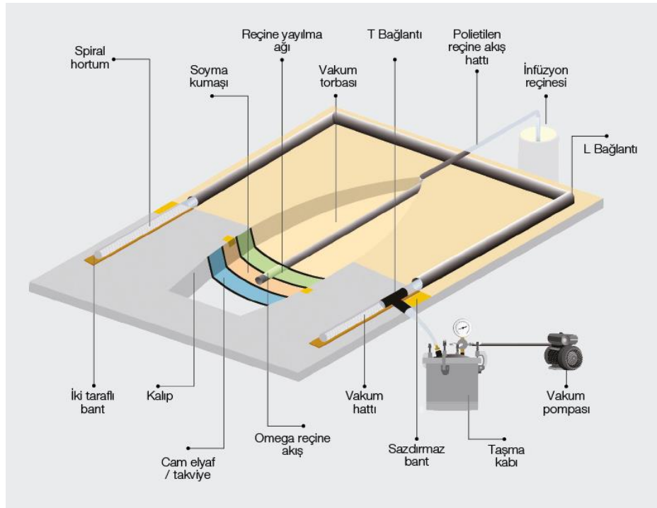
Şekil 2.11. Vakum İnfüzyon Yöntemi (Poliya)
