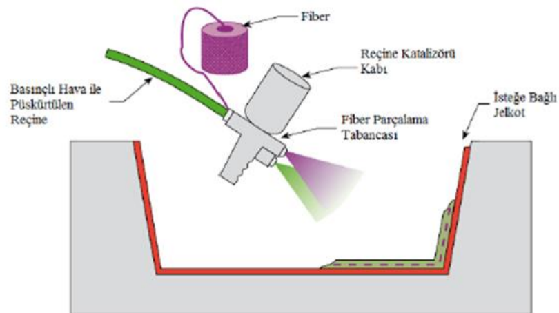
Şekil 2.7. El yatırması yöntemi
