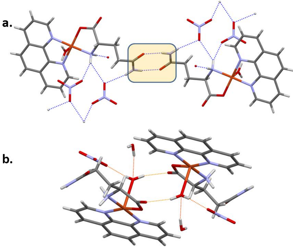
Şekil 4.13. \{[\text{Cu}(\text{phen})(\text{gln})(\text{H}_2\text{O})]\text{NO}_3 \cdot \text{H}_2\text{O}\}_n kompleksinde molekül içi a) N—H...O ve b) O—H...O hidrojen bağı etkileşimleri
