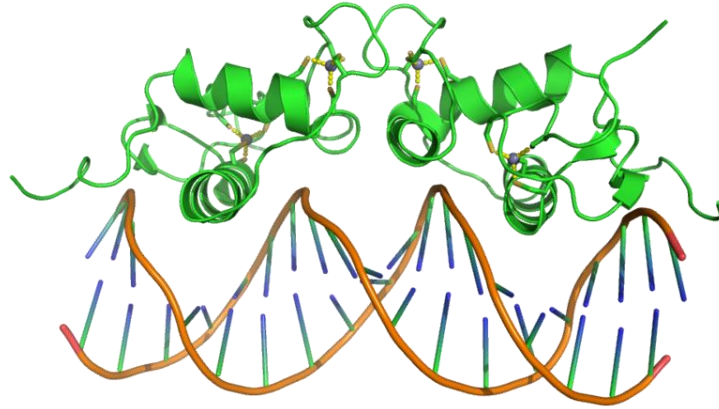
Şekil 2.11. DNA sarmalında meydana gelen major oluk bağlayıcı
