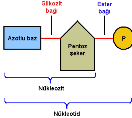
Şekil 2.6. Nükleotitin açık yapısı
