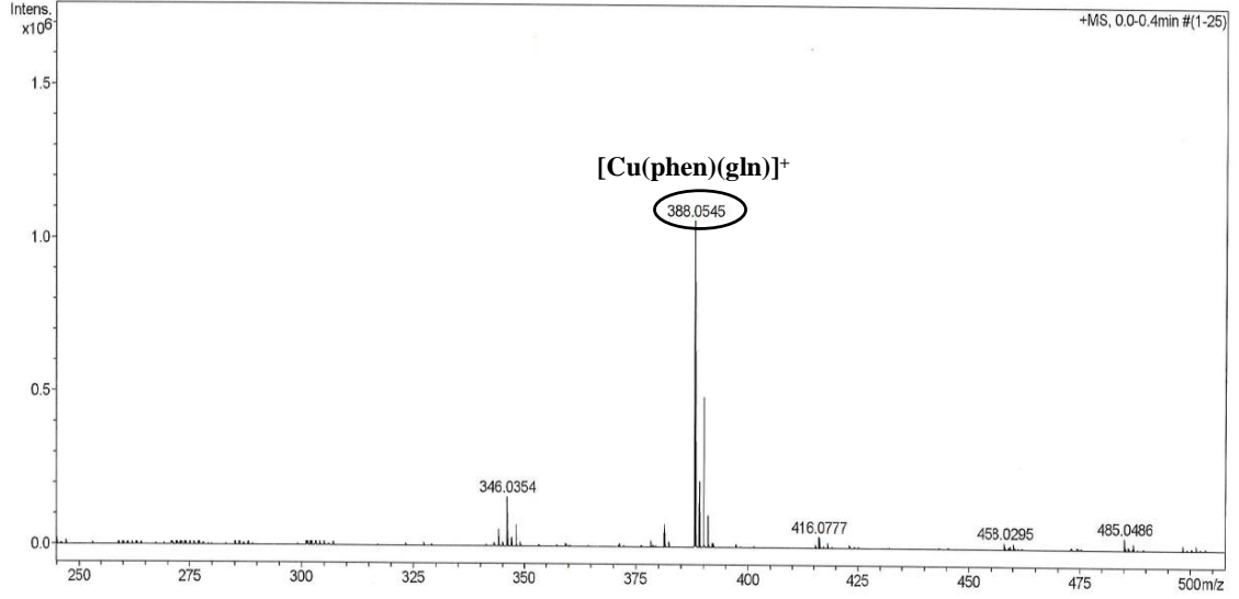
Şekil 4.10. [Cu(phen)(gln)(H 2 O)]NO 3 ·H 2 O (1) kompleksinin ESI-MS spektrumu
