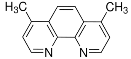
4,7-dimetil-1,10-fenantrolin (dmphen)
