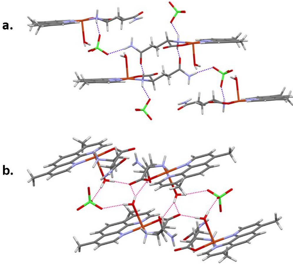
Şekil 4.15. \{[\text{Cu}(\text{dmphen})(\text{gln})(\text{H}_2\text{O})]\text{ClO}_4\}_n kompleksinde molekül içi a) N—H...O ve b) O—H...O hidrojen bağı etkileşimleri
