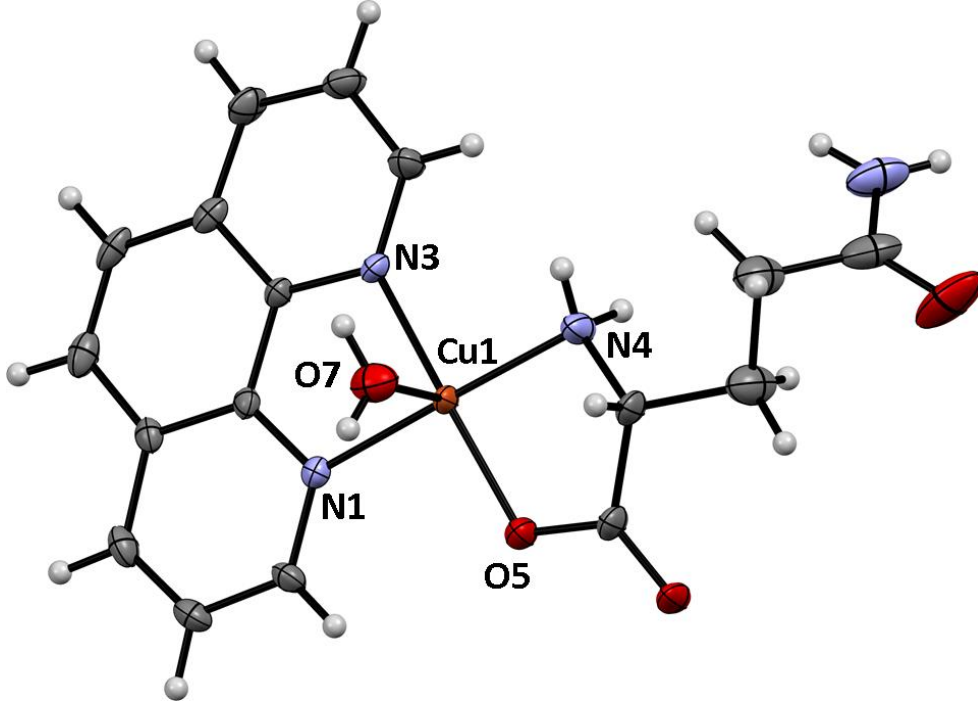
Şekil 4.12. {[Cu(phen)(gln)(H 2 O)]NO 3 ·H 2 O} n kompleksinin tek kristal X-ışını kırınım yöntemi ile aydınlatılan molekül yapısı. Koordine olmayan nitrat anyonu, kristal örgü su molekülü ve H atomları yapıyı daha iyi gösterebilmek için şekilde belirtilmemiştir. Termal titreşim elipsoidleri %30 olasılıkla verilmiştir. (Simetri kodları: (i): x+1/2, -y+1/2, -z+1 (ii): x-1/2, -y+1/2, -z+1).
