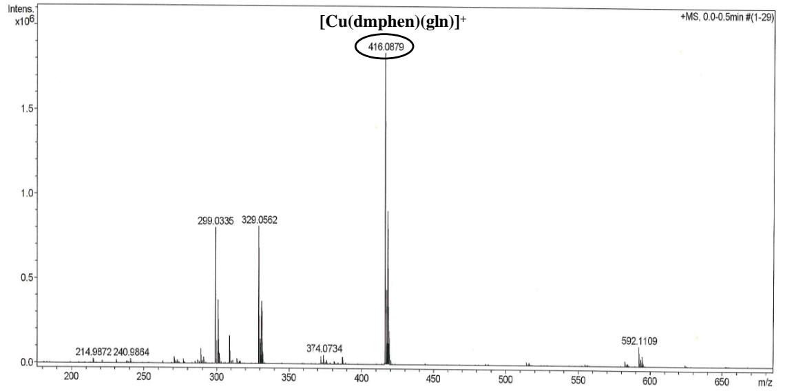
Şekil 4.11. [Cu(dmphen)(gln)(H 2 O)]ClO 4 (2) kompleksinin ESI-MS spektrumu
