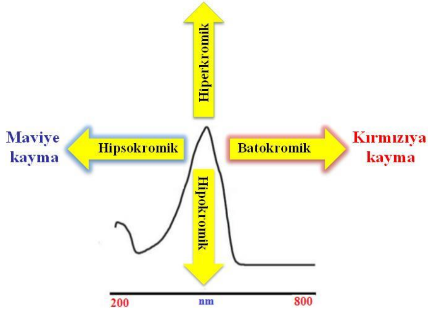
Şekil 4.16. Kompleks-DNA etkileşimlerinde, UV-spektrumunda görülen değişimler
