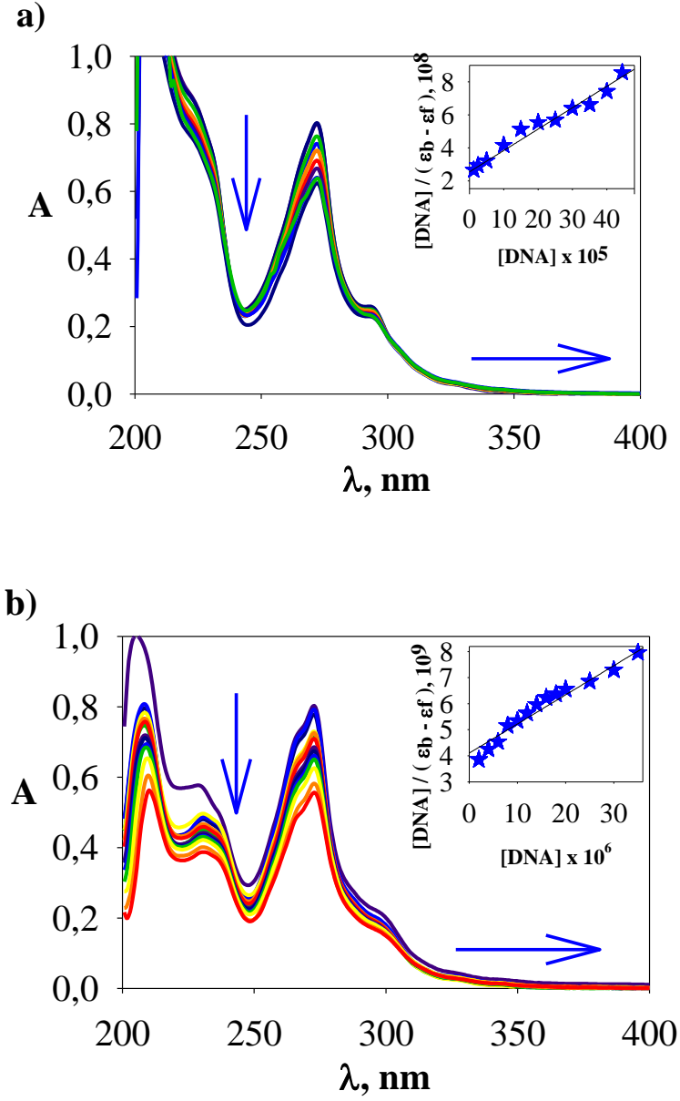
Şekil 4.17. Kompleks ve CT-DNA içeren çözeltilerin absorpsiyon spektrumları; a) Kompleks 1: \{[Cu(phen)(gln)(H_2O)]NO_3 \cdot H_2O\}_n ve b) Kompleks 2: \{[Cu(dmphen)(gln)(H_2O)]ClO_4\}_n
