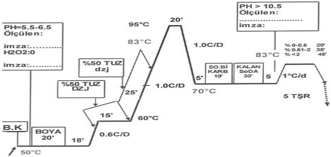
Şekil 3.5. Visikon ve Umorfil içerikli kumaşların boyama grafiği
