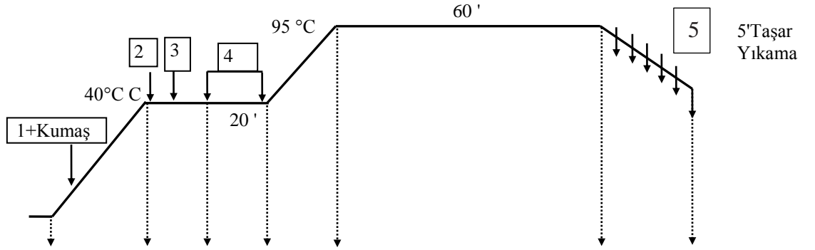
Şekil 3.2. Numune kumaşların ağartma işlem grafiği
