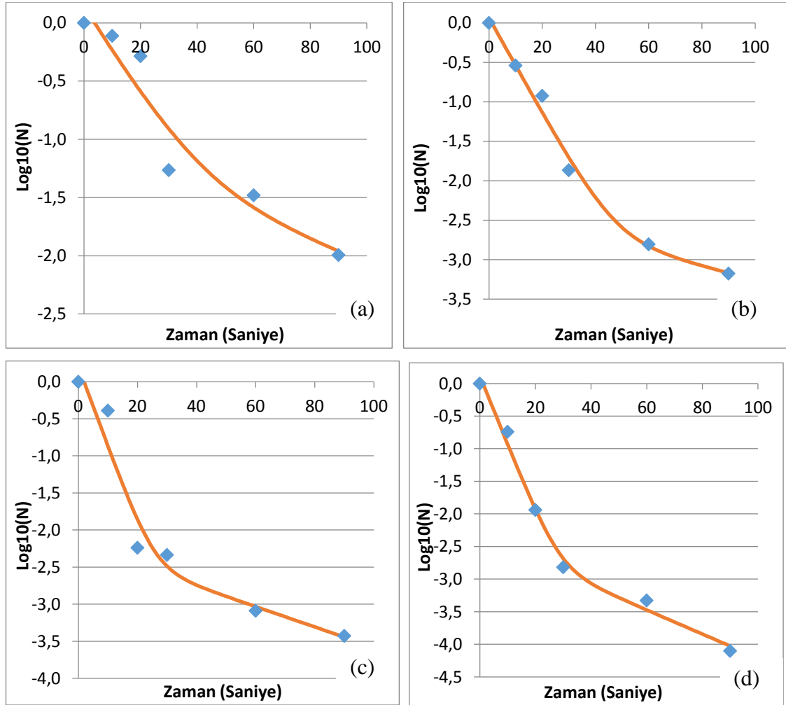
Şekil 4. 36. P. aeruginosa bakterisinin alkali ortam ile sülfat aktivasyonu prosesiyle dezenfeksiyonu sonrasında Bifazik modele göre oluşturulan inaktivasyon eğrileri (Sülfat radikalleri K_2S_2O_8 (2 mmol/L) kullanılarak elde edilmiştir. Alkali ortam için (a)0,25 mmol/L, (b)0,5 mmol/L,(c) 0,75 mmol/L, (d) 1,5 mmol/L NaOH kullanılmıştır.) (♦ ölçülen, — modellenen)
