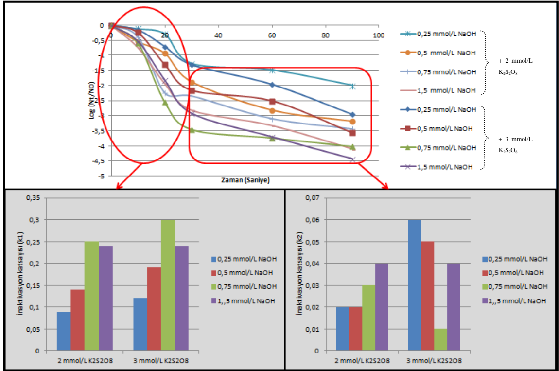
Őekil 4. 40. Alkali ortam aktivasyonu prosesinin P. aeruginosa bakterisi zerine logaritmik bakteri giderimi ve k_1 ve k_2 katsayılarının birlikte deęerlendirilmesi
