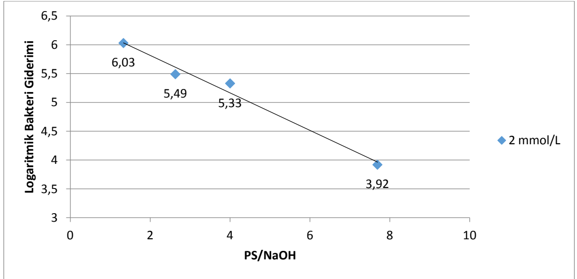
Şekil 4. 10. Alkali ortam aktivasyonu prosesinde PS(2 mmol/L)/NaOH oranlarının E. coli inaktivasyonuna etkisi
