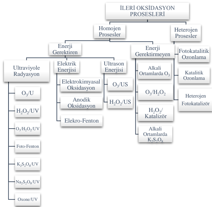
Şekil 2. 1. İleri Oksidasyon Prosesleri
