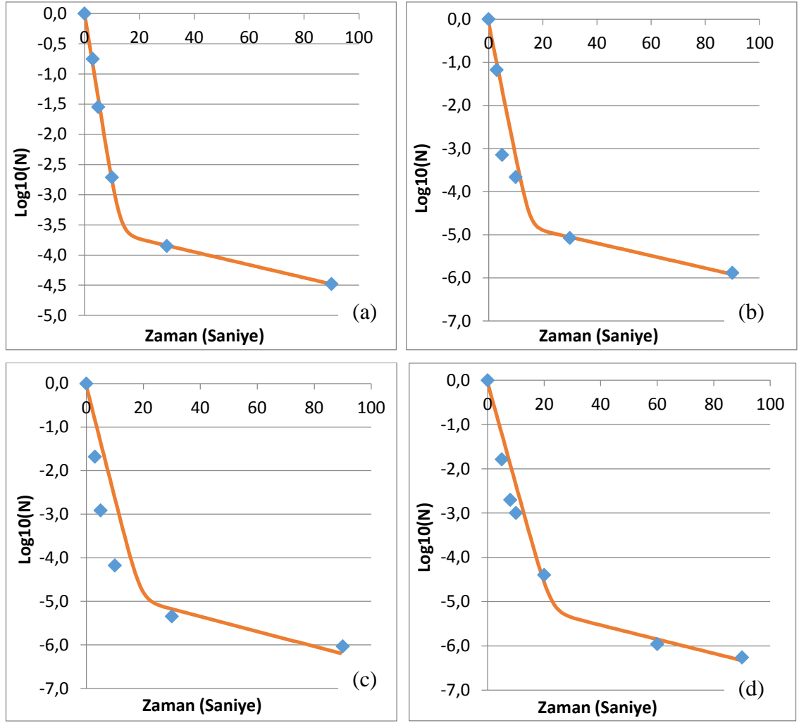
Şekil 4. 32. E. coli bakterisinin alkali ortam ile sülfat aktivasyonu prosesiyle dezenfeksiyonu sonrasında Bifazik modele göre oluşturulan inaktivasyon eğrileri (Sülfat radikalleri K_2S_2O_8 (3 mmol/L) kullanılarak elde edilmiştir. Alkali ortam için (a)0,25 mmol/L, (b)0,5 mmol/L,(c) 0,75 mmol/L, (d) 1,5 mmol/L NaOH kullanılmıştır.) ( ◆ ölçülen, — modellenen)
