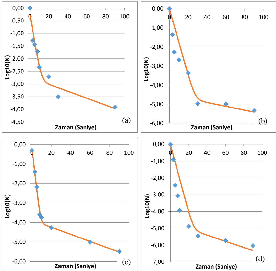
Şekil 4. 31. E. coli bakterisinin alkali ortam ile sülfat aktivasyonu prosesiyle dezenfeksiyonu sonrasında Bifazik modele göre oluşturulan inaktivasyon eğrileri (Sülfat radikalleri K_2S_2O_8 (2 mmol/L) kullanılarak elde edilmiştir. Alkali ortam için (a)0,25 mmol/L, (b)0,5 mmol/L,(c) 0,75 mmol/L, (d) 1,5 mmol/L NaOH kullanılmıştır.) (♦ ölçülen, — modellenen)
