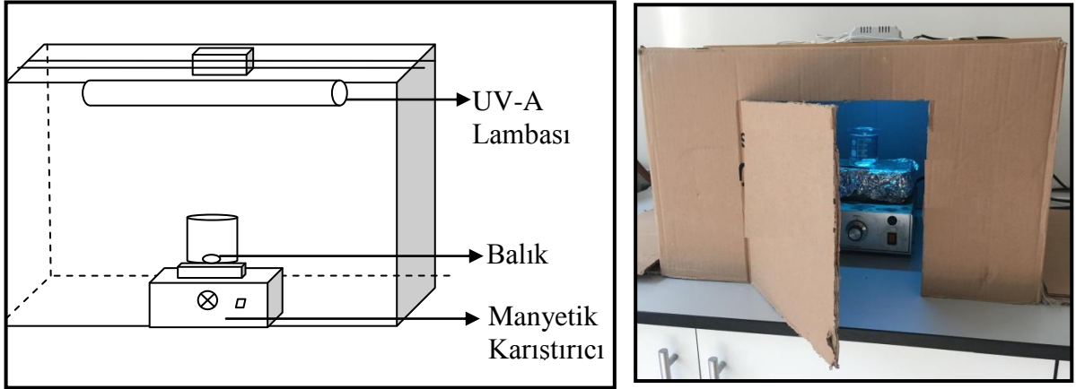
Şekil 3. 1. Laboratuar ölçekli UV-A Reaktörü
