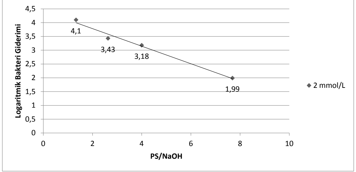
Şekil 4. 16. Alkali ortam aktivasyonu prosesinde PS(2 mmol/L)/NaOH oranlarının P. aeruginosa inaktivasyonuna etkisi
