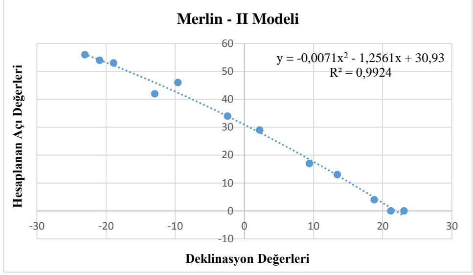
Şekil 4.56. Polimetrik Merlin - II modelin deklinaşyon eęrisi – Hatay
