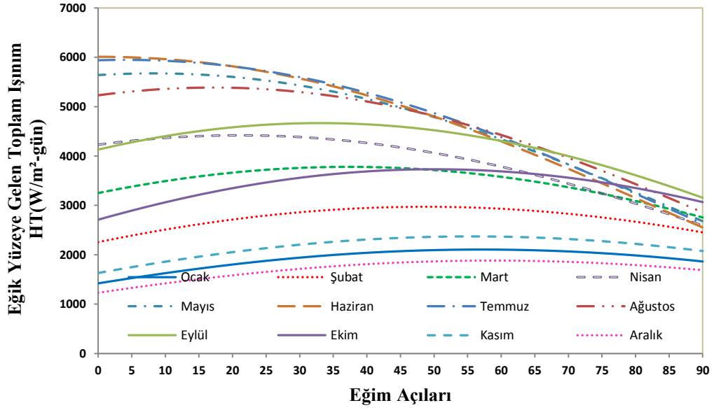
Şekil 4.36. Sinop için yıllık optimum açığa göre güneş ışınım değerleri
