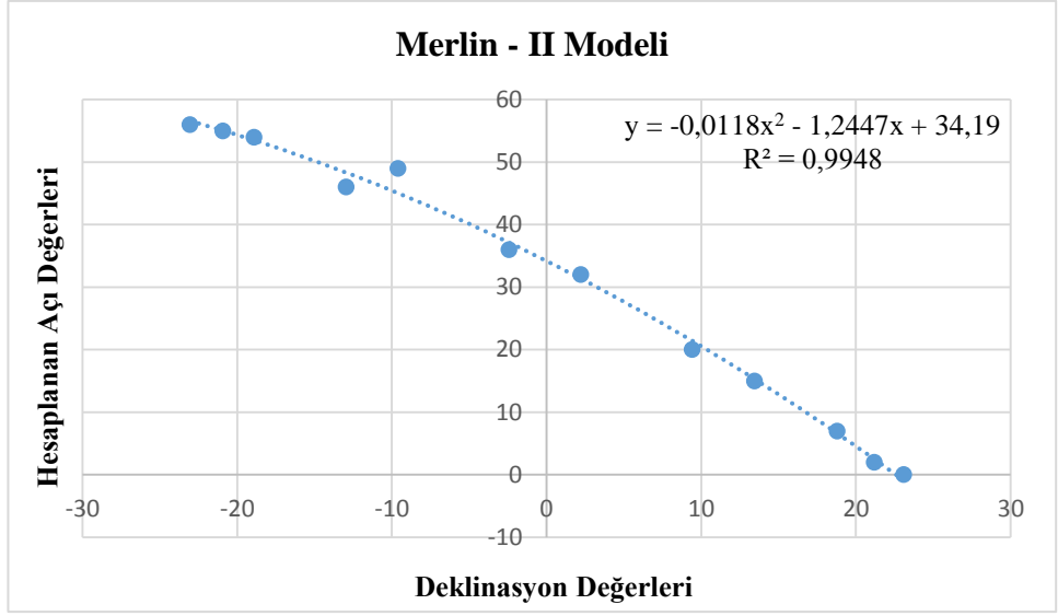
Şekil 4.50. Polimetrik Merlin - II modelin deklinasyon eğrisi – Erzurum
