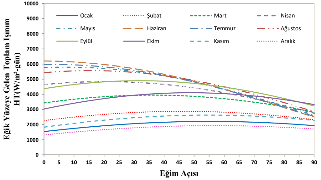
Şekil 4.6. Bursa için yıllık optimum açığa göre güneş ışınım değerleri
