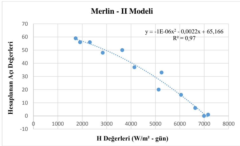
Şekil 4.116. Polimetrik Merlin - II modelin H eğrisi – Van
