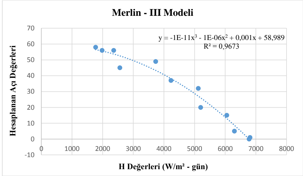
Şekil 4.108. Polimetrik Merlin - III modelin H eğrisi – Konya
