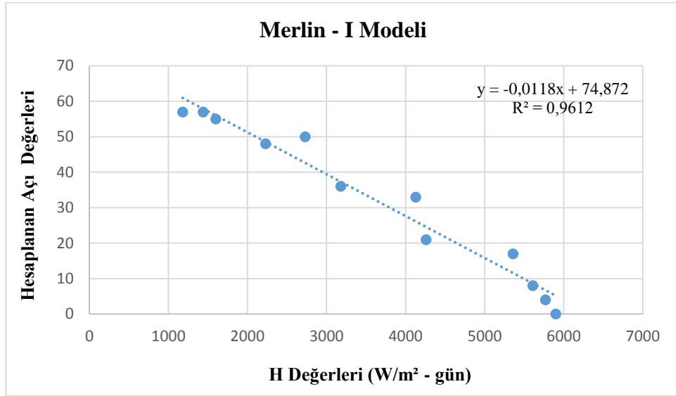
Şekil 4.85. Linear Merlin - I modelinin H eğrisi – Edirne
