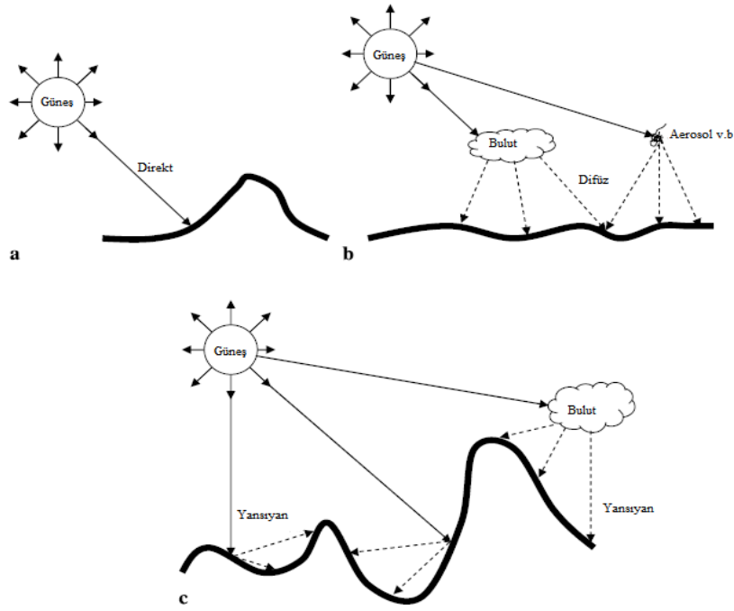
Şekil 2.2. Yeryüzüne gelen güneş ışınımının dağılımı
