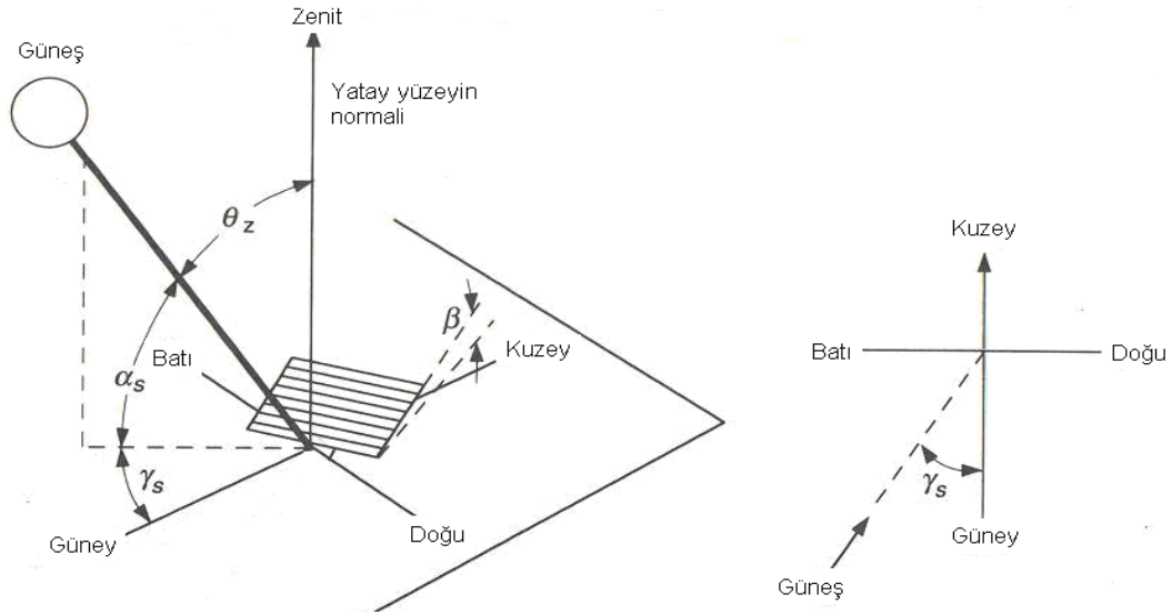
Şekil 2.13. Güneşle ilgili açıların birbirleri ile ilişkileri
