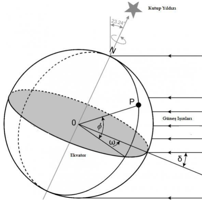
Şekil 2.6. Enlem ( \phi ), saat ( \omega ) ve deklinasyon açıları ( \delta )
