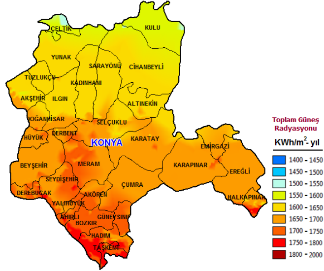
Şekil 3.19. Konya güneş ışınımı yoğunluğunun ilçelere göre dağılımı (Anonim 2018)
