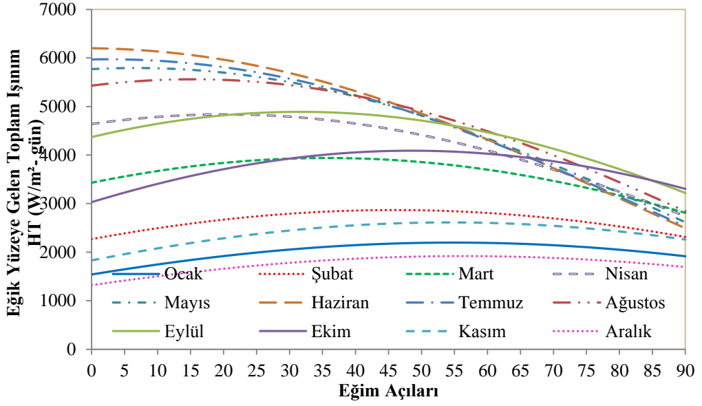
Şekil 4.12. Erzurum için yıllık optimum açığa göre güneş ışınlam değerleri
