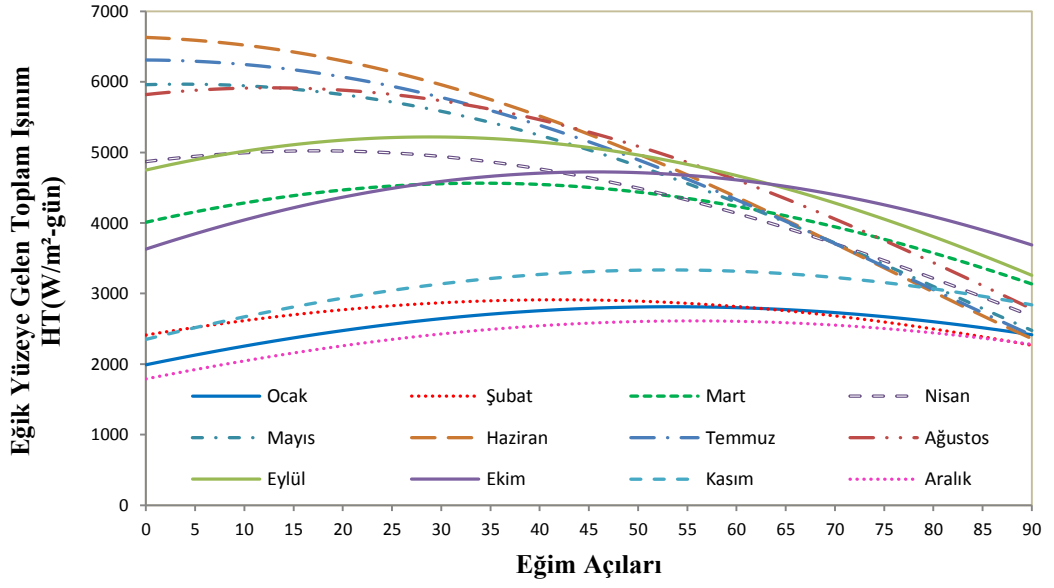
Şekil 4.18. Hatay için yıllık optimum açığa göre güneş ışınım değerleri
