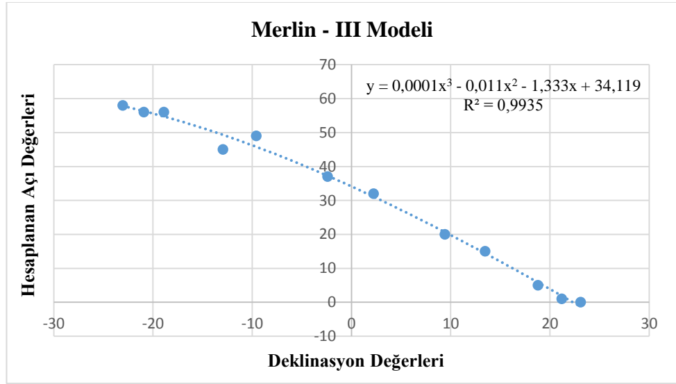
Şekil 4.69. Polimetrik Merlin - III modelin deklinasyon eğrisi – Konya
