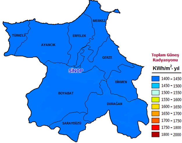
Şekil 3.23. Sinop güneş ışınımı yoğunluğunun ilçelere göre dağılımı (Anonim 2018n)
