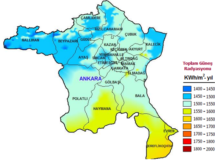
Şekil 3.1. Ankara güneş ışınımı yoğunluğunun ilçelere göre dağılımı (Anonim 2018d)
