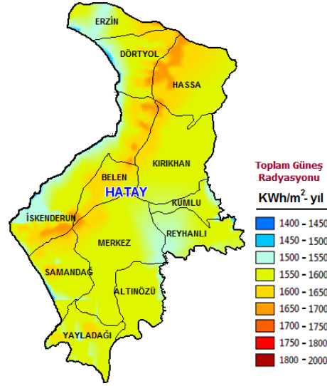
Şekil 3.11. Hatay güneş ışınımı yoğunluğunun ilçelere göre dağılımı (Anonim 2018)
