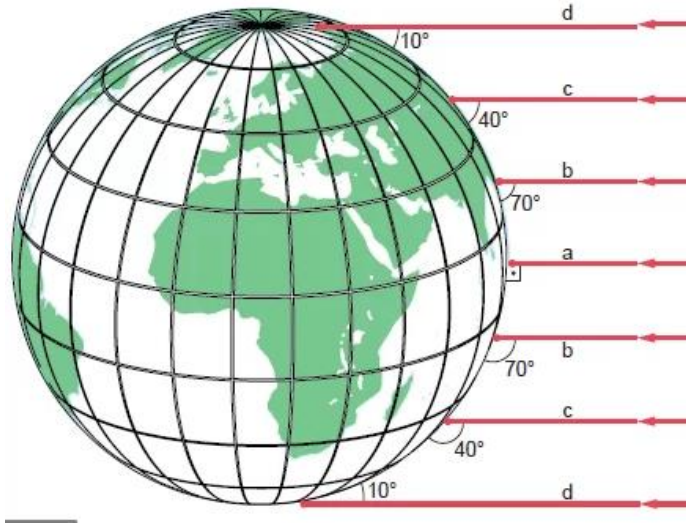
Şekil 2.14. Güneş geliş ışınlarının dünya üzerinde aldığı açısal değerleri
