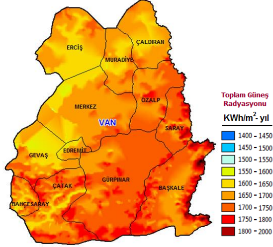
Şekil 3.25. Van güneş ışınımı yoğunluğunun ilçelere göre dağılımı (Anonim 2018o)
