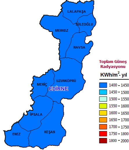
Şekil 3.5. Edirne güneş ışınımı yoğunluğunun ilçelere göre dağılımı (Anonim 2018f)
