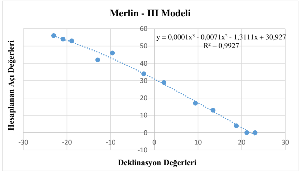
Şekil 4.57. Polimetrik Merlin - III modelin korelasyon eęrisi – Hatay
