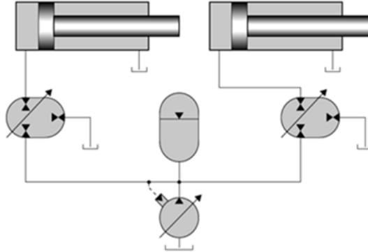
Şekil 16: Akümlatör kullanılan basınç dengeli hidrolik devre (Raymond ve Chenoweth 1993)
