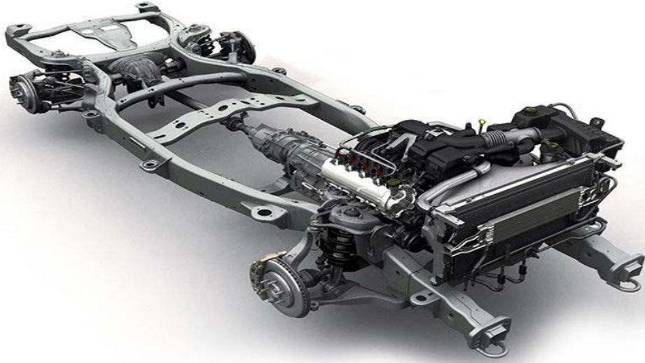
Şekil 2.2. İçten yanmalı motor teknolojisine sahip araç şasisi (Carstechnic 2018)
