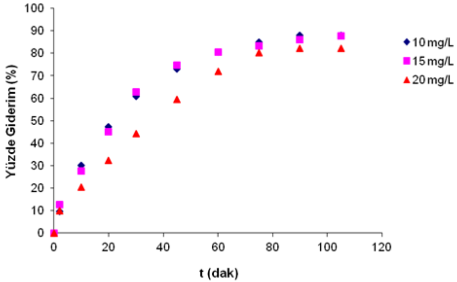
Şekil 4.15. Farklı derişimlerdeki BY için zamana karşı yüzde giderim deęişimi
