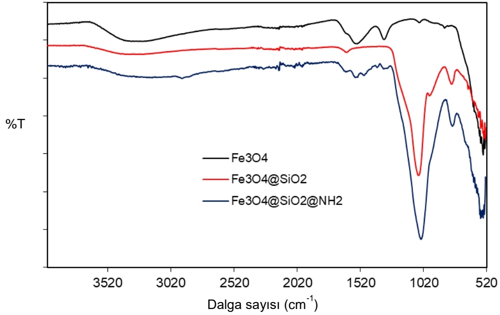
Şekil 4.3. \text{Fe}_3\text{O}_4 , \text{Fe}_3\text{O}_4@\text{SiO}_2 ve \text{Fe}_3\text{O}_4@\text{SiO}_2@\text{NH}_2 ' nin FT-IR spektrumları
