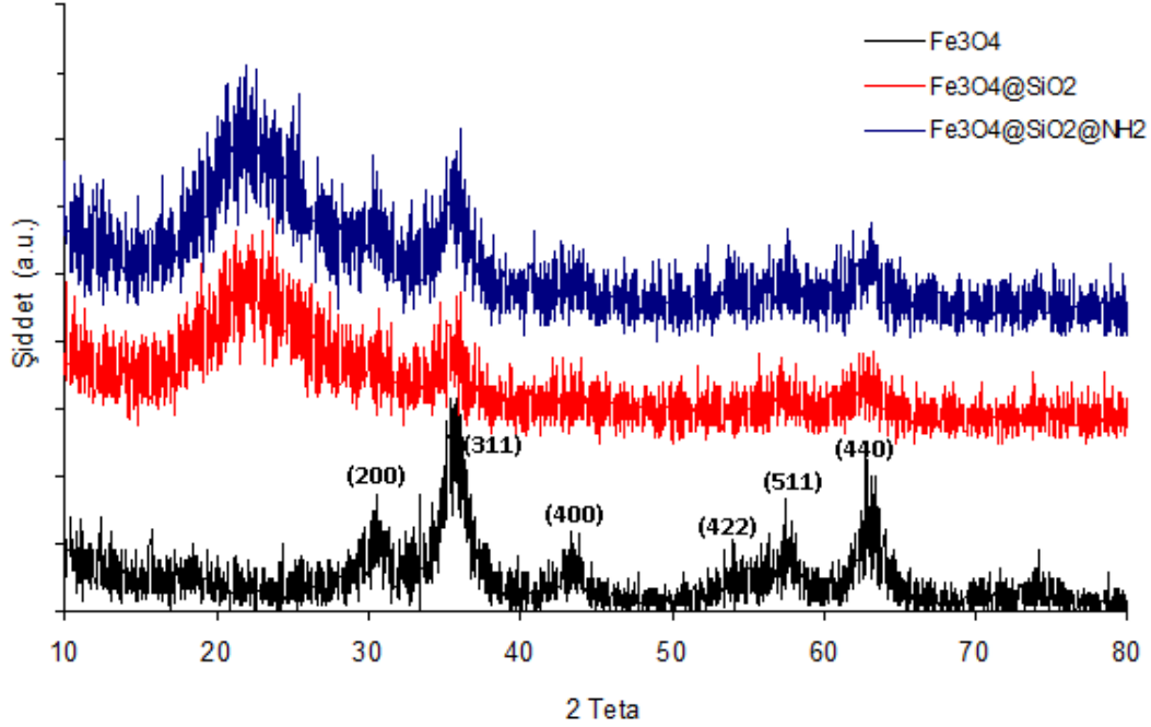
Şekil 4.4. Fe_3O_4 , Fe_3O_4@SiO_2 ve Fe_3O_4@SiO_2@NH_2 ' nin XRD spektrumları
