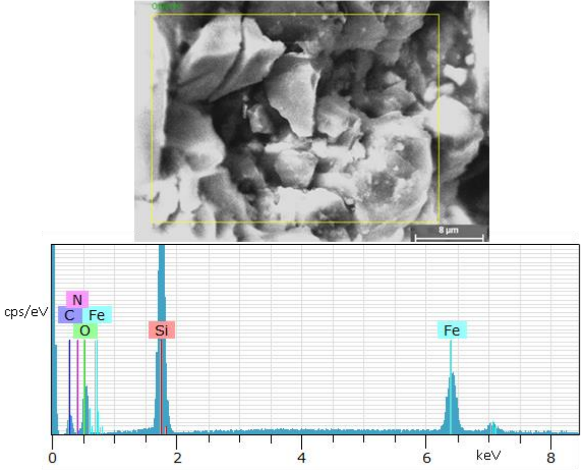
Şekil 4.2. \text{Fe}_3\text{O}_4@\text{SiO}_2@\text{NH}_2 ' nin SEM/EDX analizi
