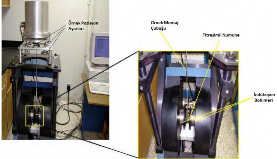
Şekil 2.18. Bir VSM cihazının fotoğrafı (Dunn 2006)
