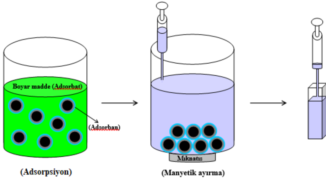
Şekil 3.1. Süperparamanyetik Fe 3 O 4 nanopartiküllerinin sentezi, SiO 2 ile kaplanması, -NH 2 grubu ile fonksiyonelleştirilmesi ve boyar madde adsorpsiyonu
