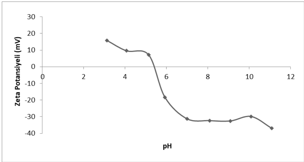
Őekil 4.7. \text{Fe}_3\text{O}_4@\text{SiO}_2@\text{NH}_2 nanokompozitinin zeta potansiyeli
