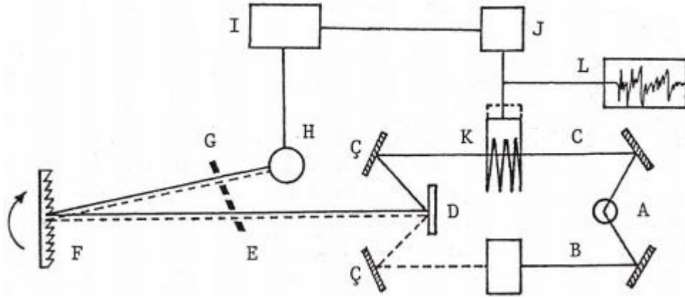
Şekil 2.14. FT-IR cihazının şematik gösterimi (Erdik 1998)
