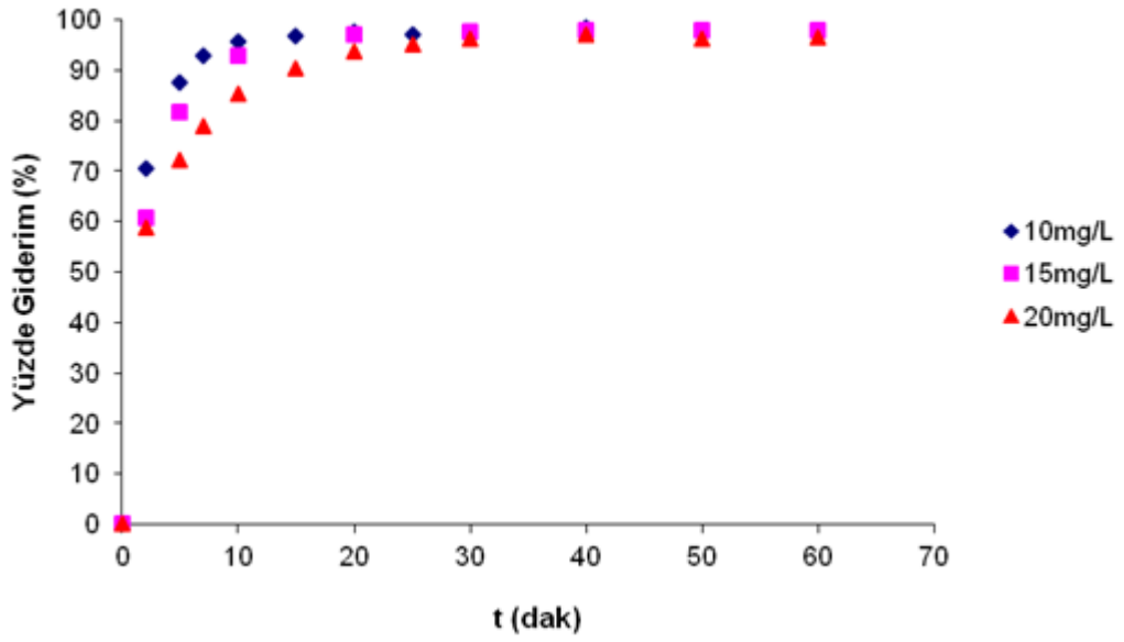
Şekil 4.14. Farklı derişimlerdeki LG için zamana karşı yüzde giderim deęişimi
