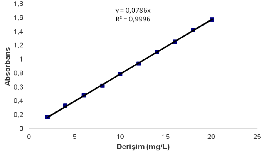
Şekil 4.8. LG boyar maddesi için kalibrasyon grafiği
