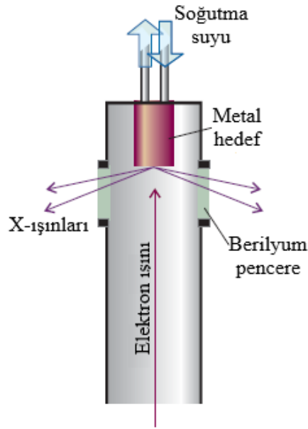
Şekil 2.10. X-ışınlarının oluşumu (Atkins ve Paulo 2006)
