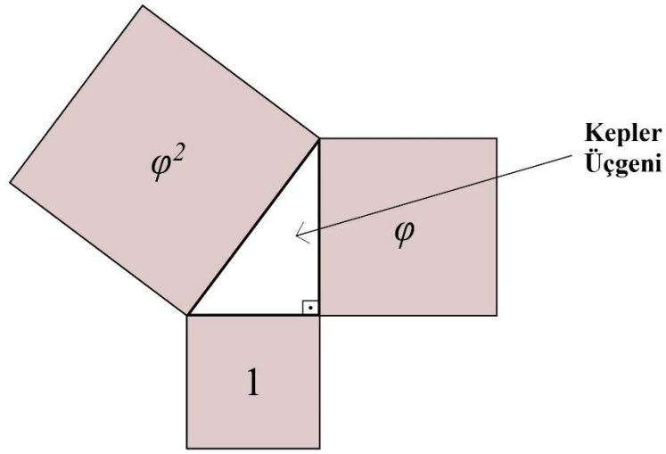
Şekil 1.1. Kepler Üçgeni
