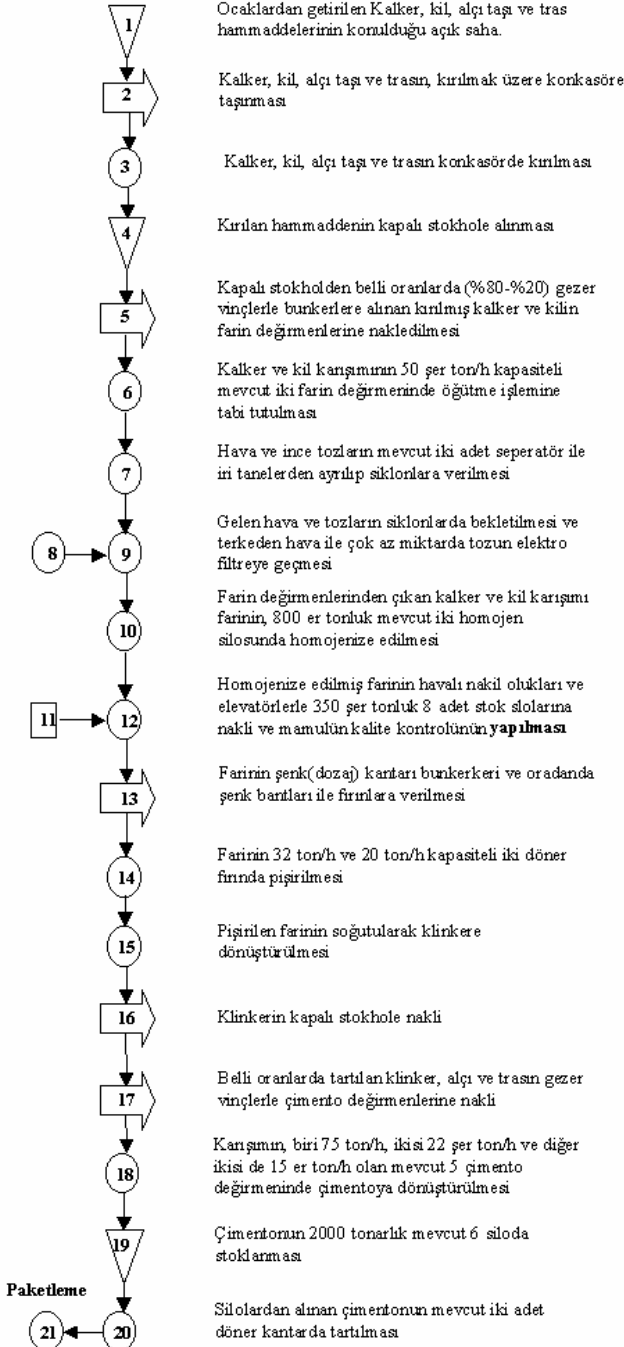
Şekil 1. İş Akım Şeması
