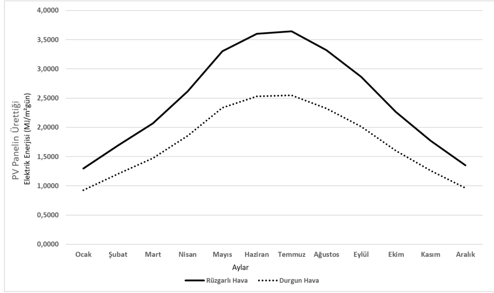
Şekil 4.8. Rüzgarın PV panelin ürettiği aylık ortalama günlük elektrik enerjisine etkisi
