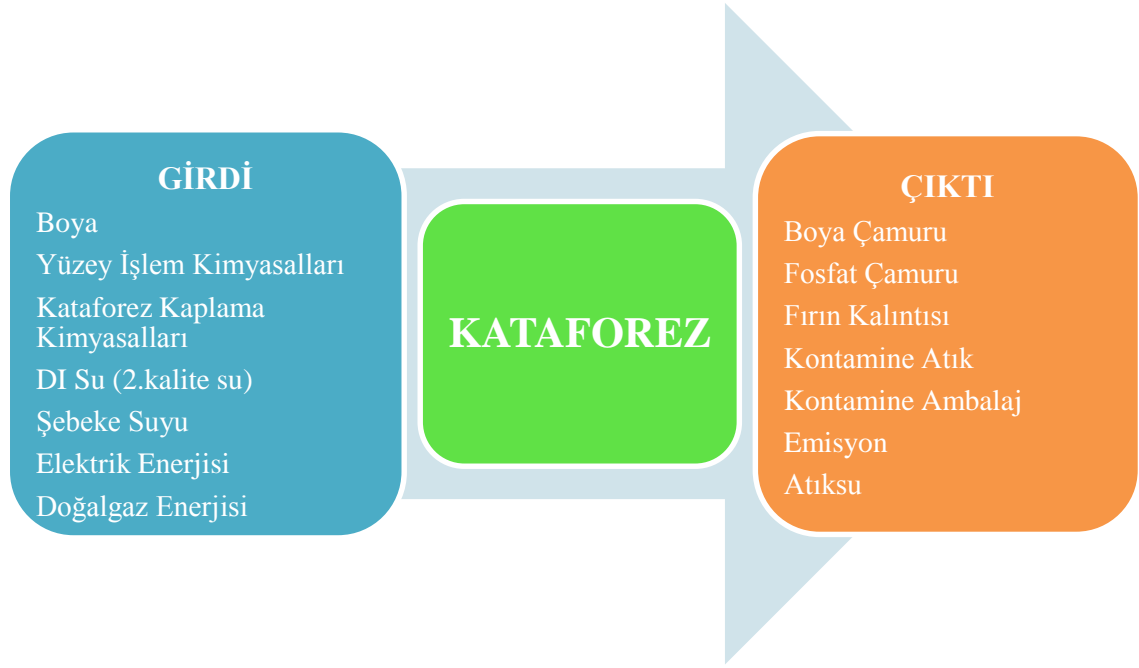
Şekil 4.1. Kataforez girdileri ve çıktıları
