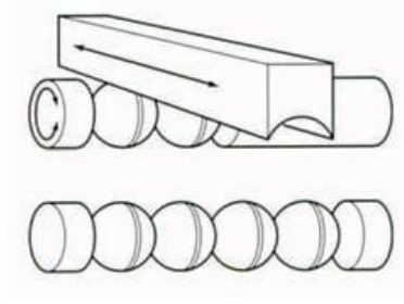
Çizim 2 - Boncuk tel eğesi.
