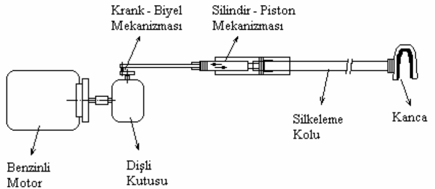
Şekil 2. Mekanik titreşimli zeytin hasat makinası
