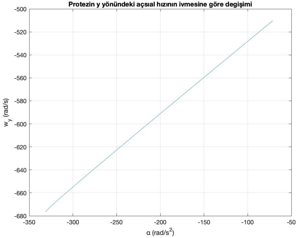
Şekil 29. (5) numaralı denklemden y yönündeki açısal hızın dinamik değişimi
