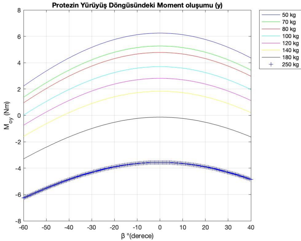
Şekil 49. Farklı vücut ağırlıklarına göre protezin y yönündeki moment değişimi
