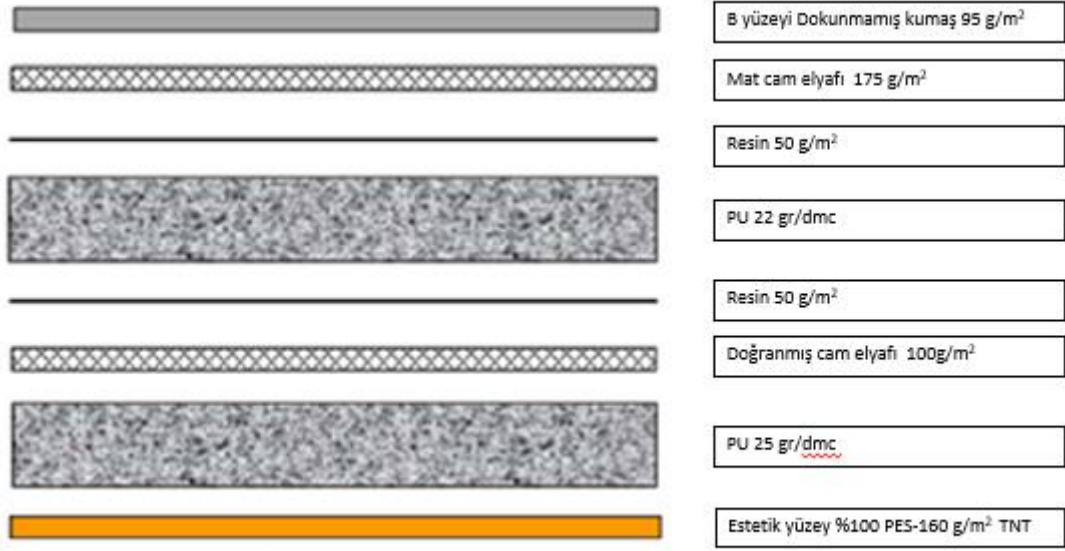
Őekil 4.3. Numune 2'in katmanları
