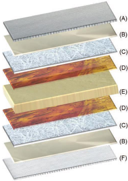
Şekil 3.1. Tavan yapısı (Silva, Calçada, & Massarelli, 2014)
