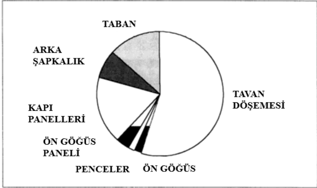
Şekil 1.2. Çeşitli iç kaplama bileşenlerinin 2000 Hz’de (koltuklar hariç) otomobilin iç kısmındaki ses yutum katkısı (Aggarwal, Khan, & Crepeau, 1998)
