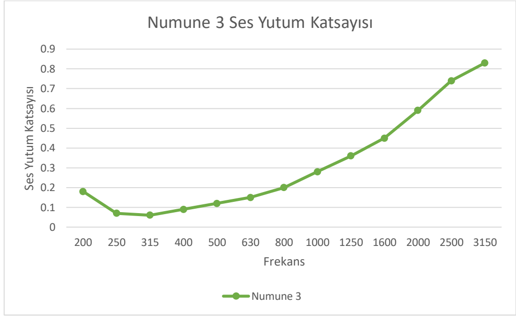
Őekil 4.10. Numune 3'ün ses yutum katsayısı lmleri
