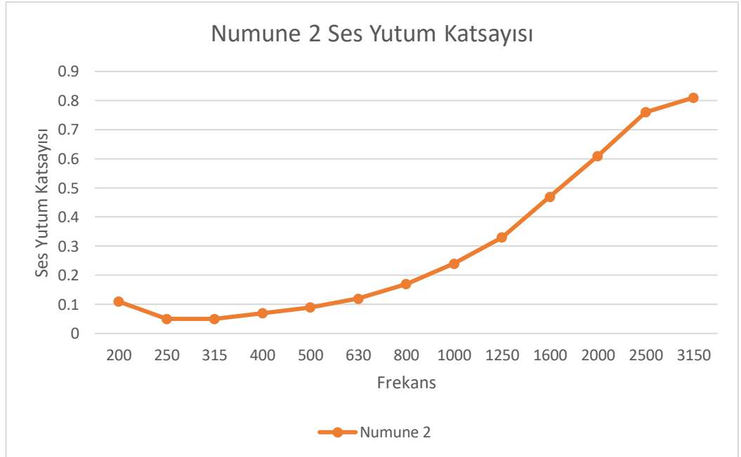
Őekil 4.9. Numune 2'nin ses yutum katsayısı lmleri
