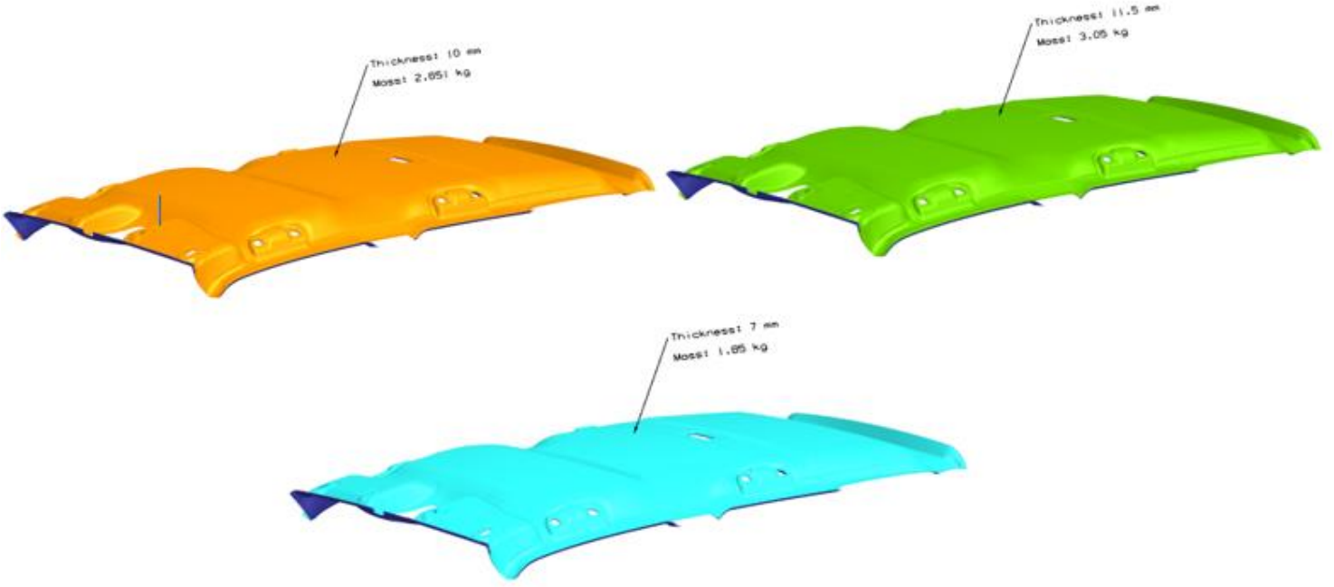
Şekil 4.13. Tasarımların ağırlık ölçümleri
