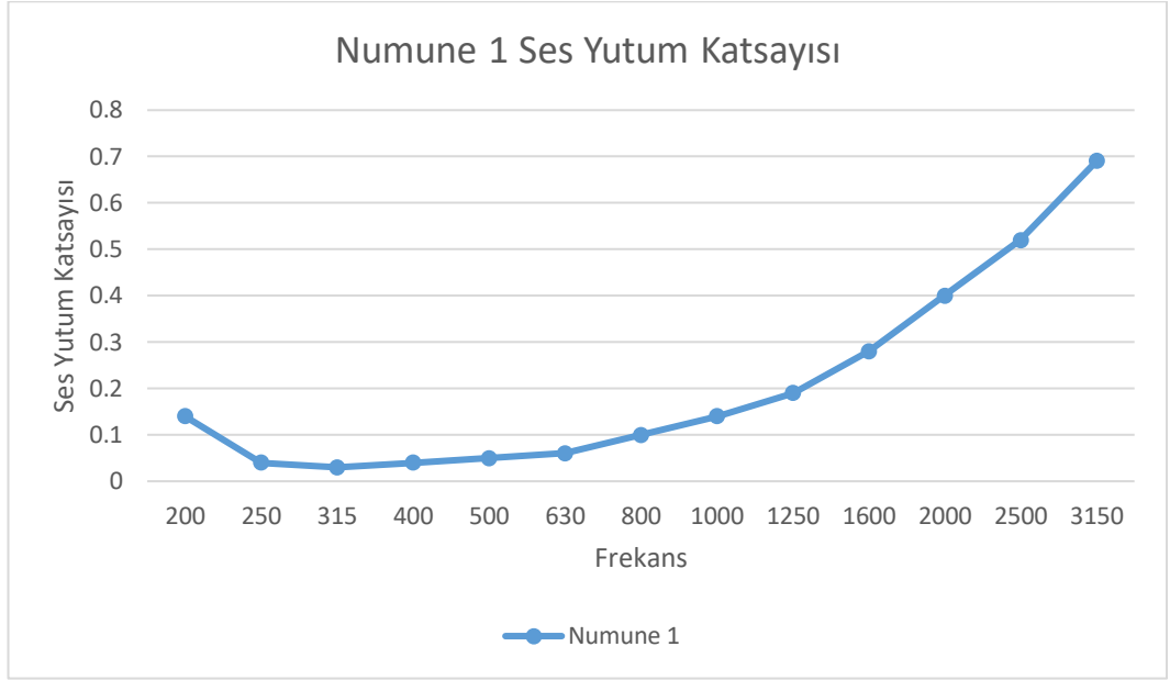
Őekil 4.8. Numune 1'in ses yutum katsayısı lmleri
