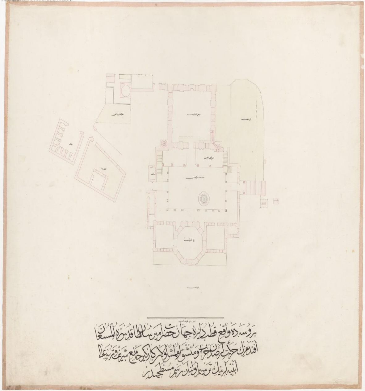
Ek 12: Depremde hasar alan Emir Sultan Cami-i Şerifi ve Türbesi Planı. (PLK.p 03443)
