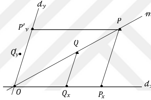
Şekil 5.2.1. P'_y P_x \parallel Q'_y Q_x
