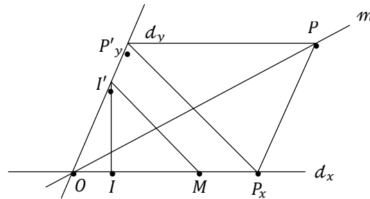
Şekil 5.2.2. I'M \parallel P'_y P_x
