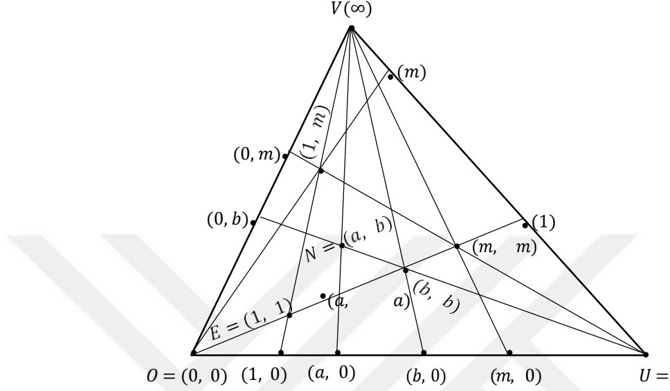
Şekil 6.2.1. Noktaların tayini
