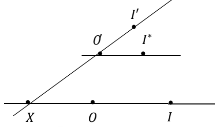
Şekil 5.1.5. d \cap m = X için (d, O, I) \cong (m, O', I') dür
