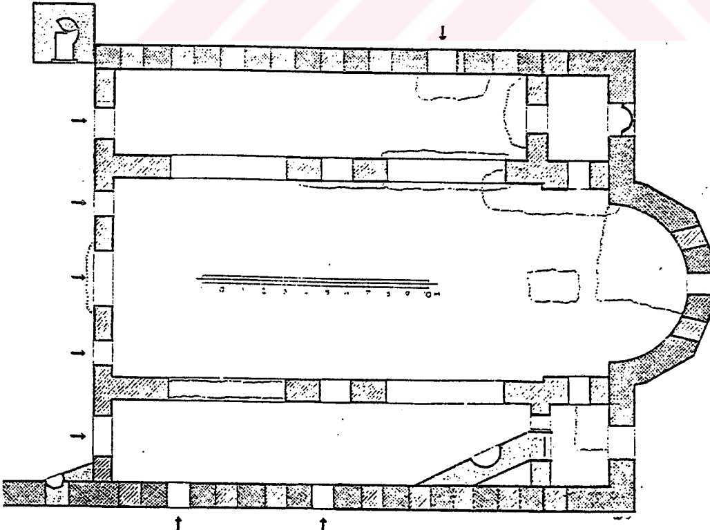
Ayasofya Kilisesi plan ve kesiti...
