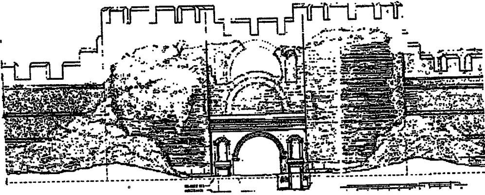
Istanbul Kapısı ve surlarının restitüsyonu
