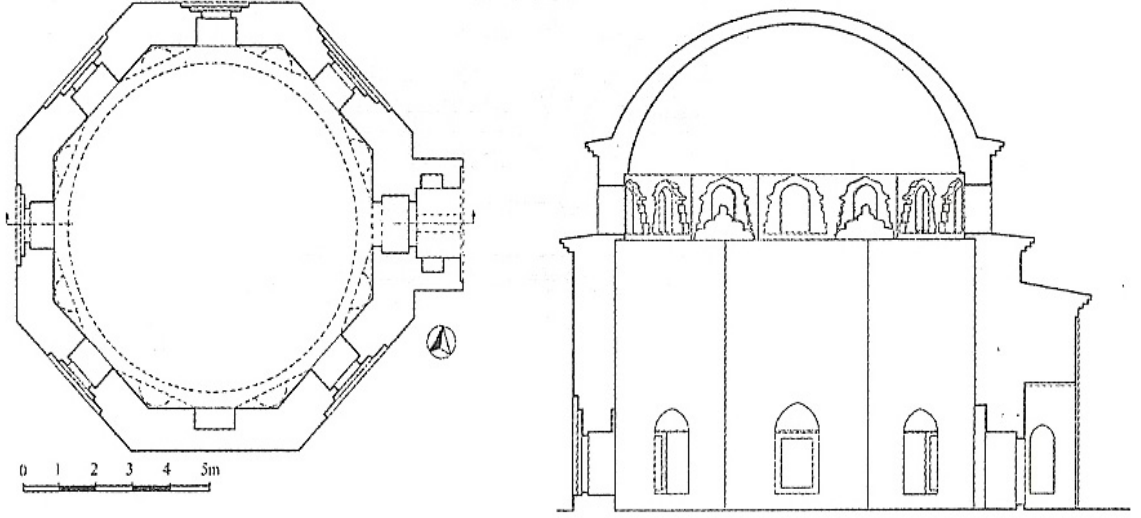
Hamza Bey Türbesi. Kesit ve plan
