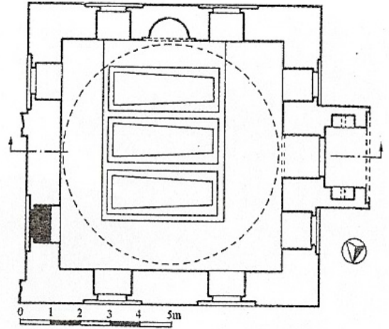
Karamustafa Paşa Türbesi. Kesit ve Plan
